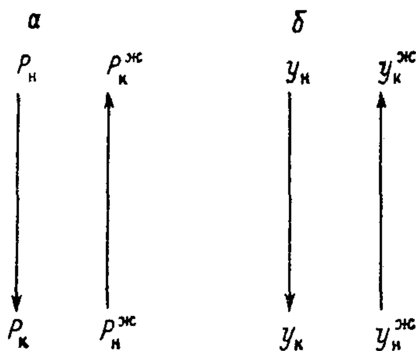
Рис. 8.4 Противоточная схема движения фаз: p — парциальные давления; y — концентрация поглощаемого газа
