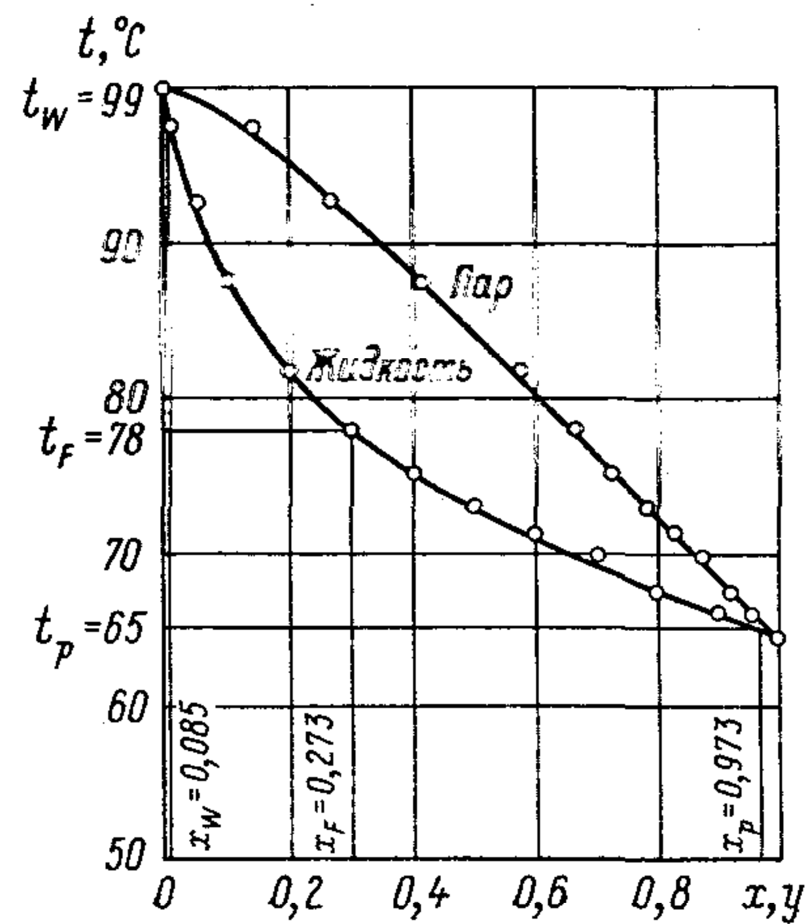
Рис. 9.9. Кривые температур кипения смеси метилового спирта и воды
