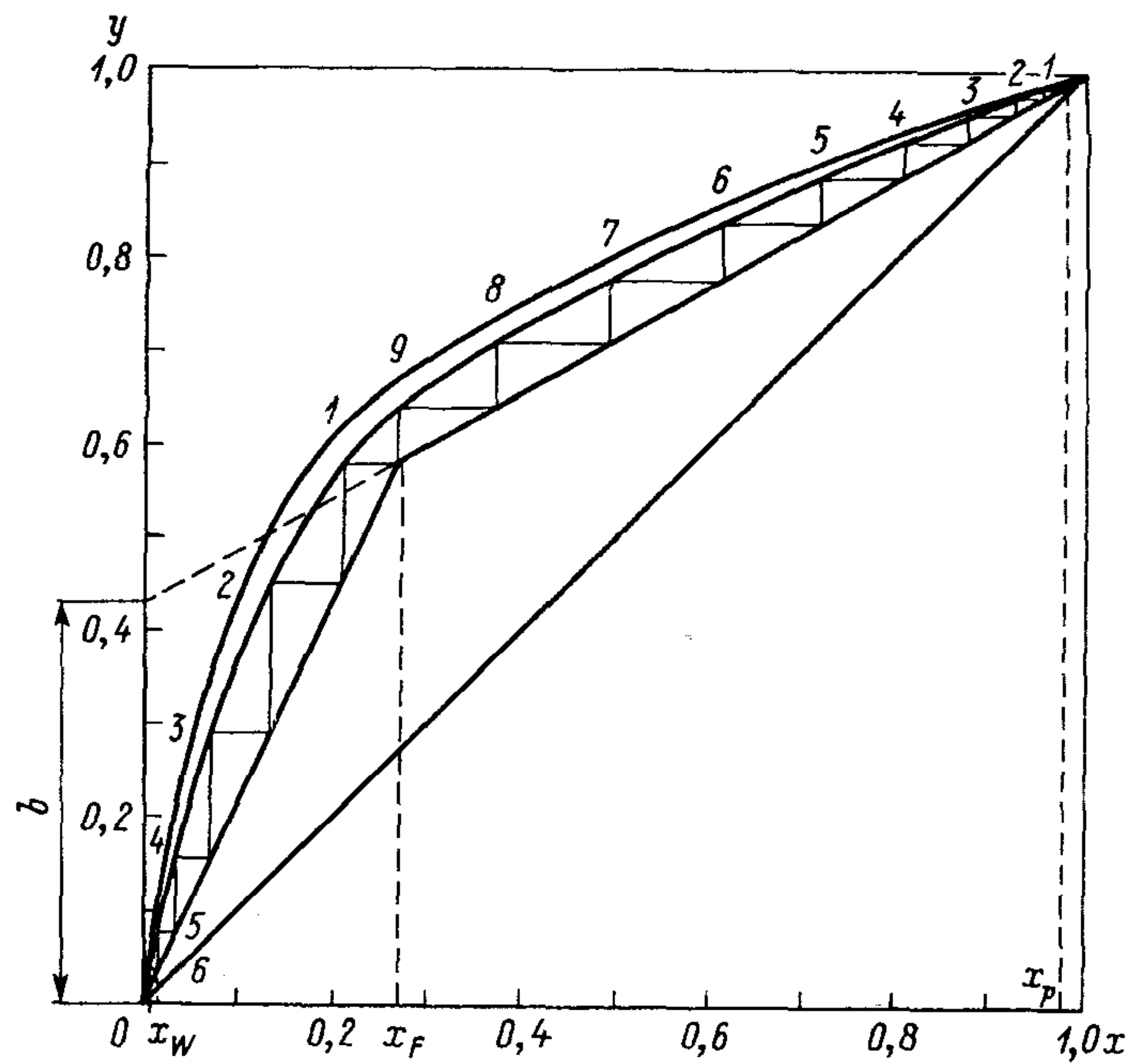
Рис. 9.6. Графическое определение числа действительных тарелок
