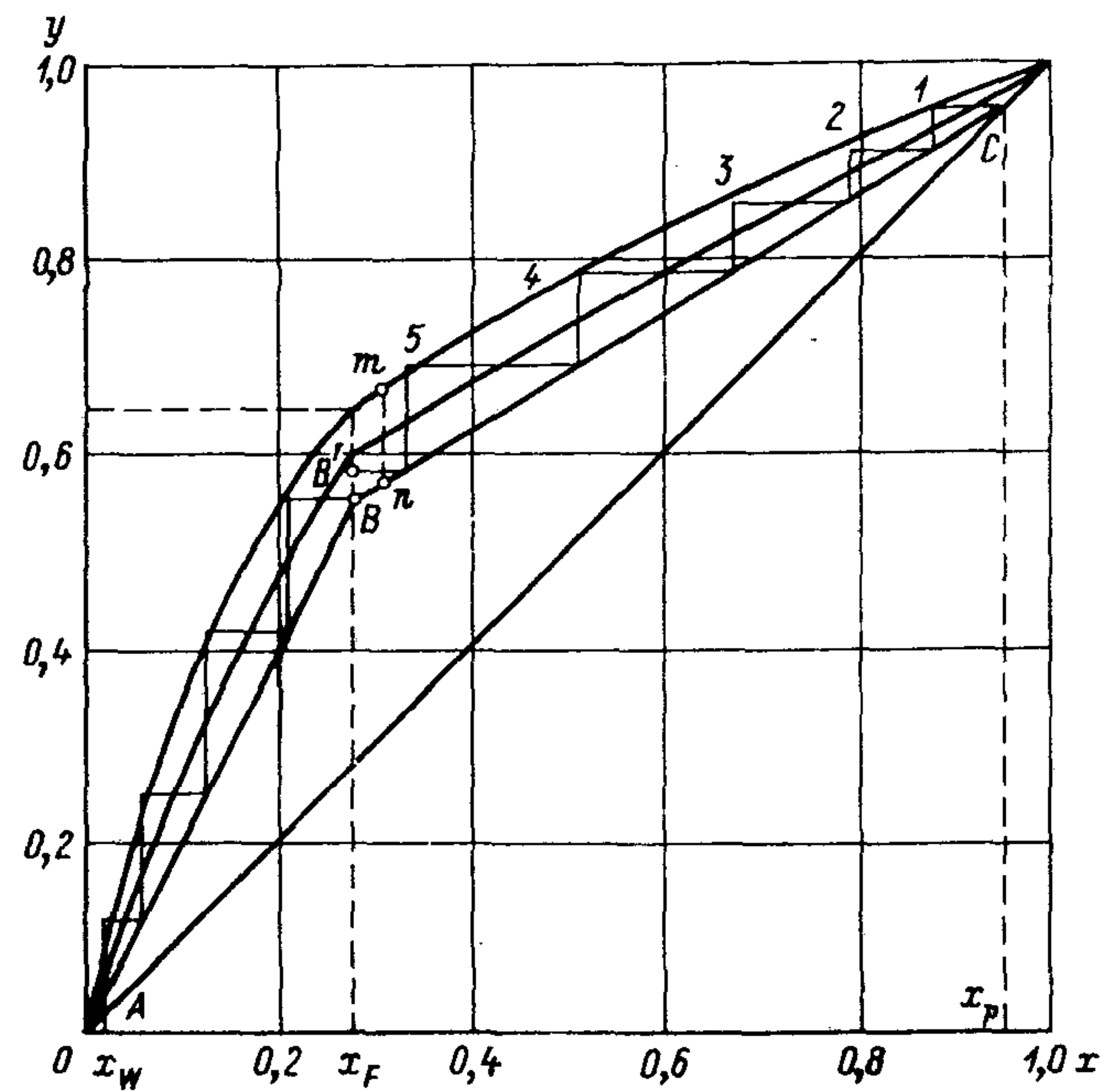
Рис. 9.7. Определение числа единиц переноса
