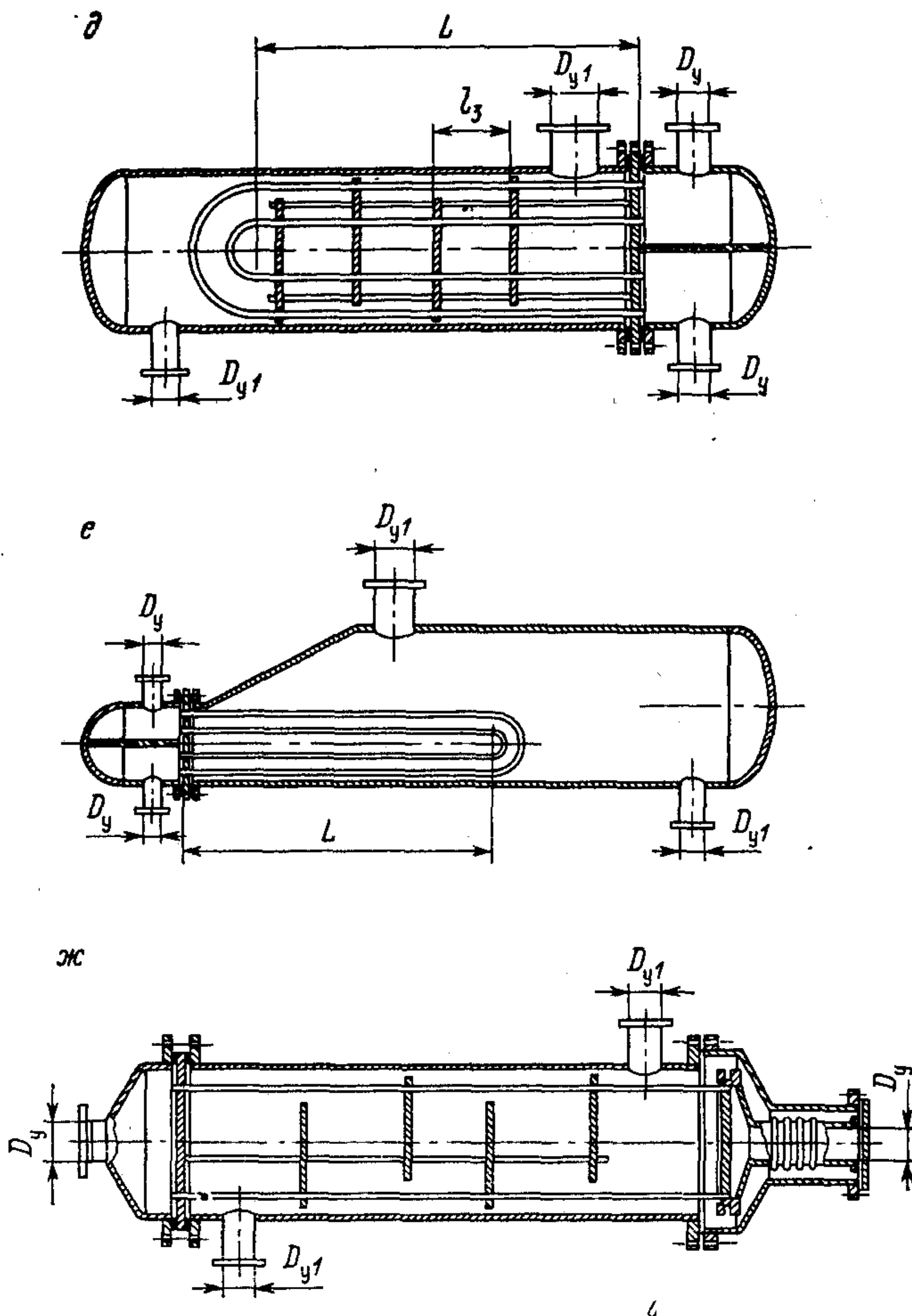
Рис. 5.9. Аппараты теплообменные кожухотрубные стальные
