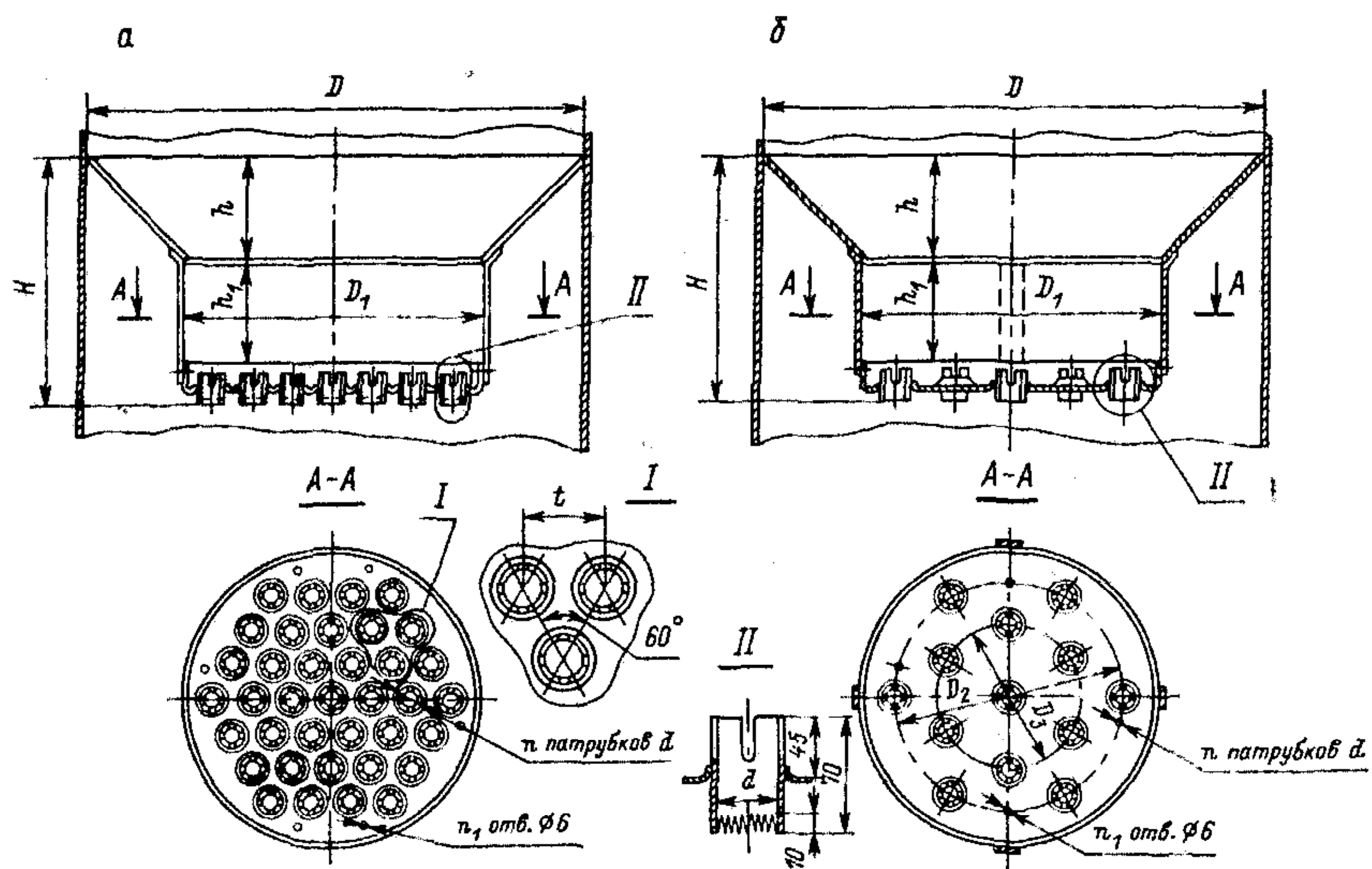
Рис. 8.15. Тарелка ТСН-2:
