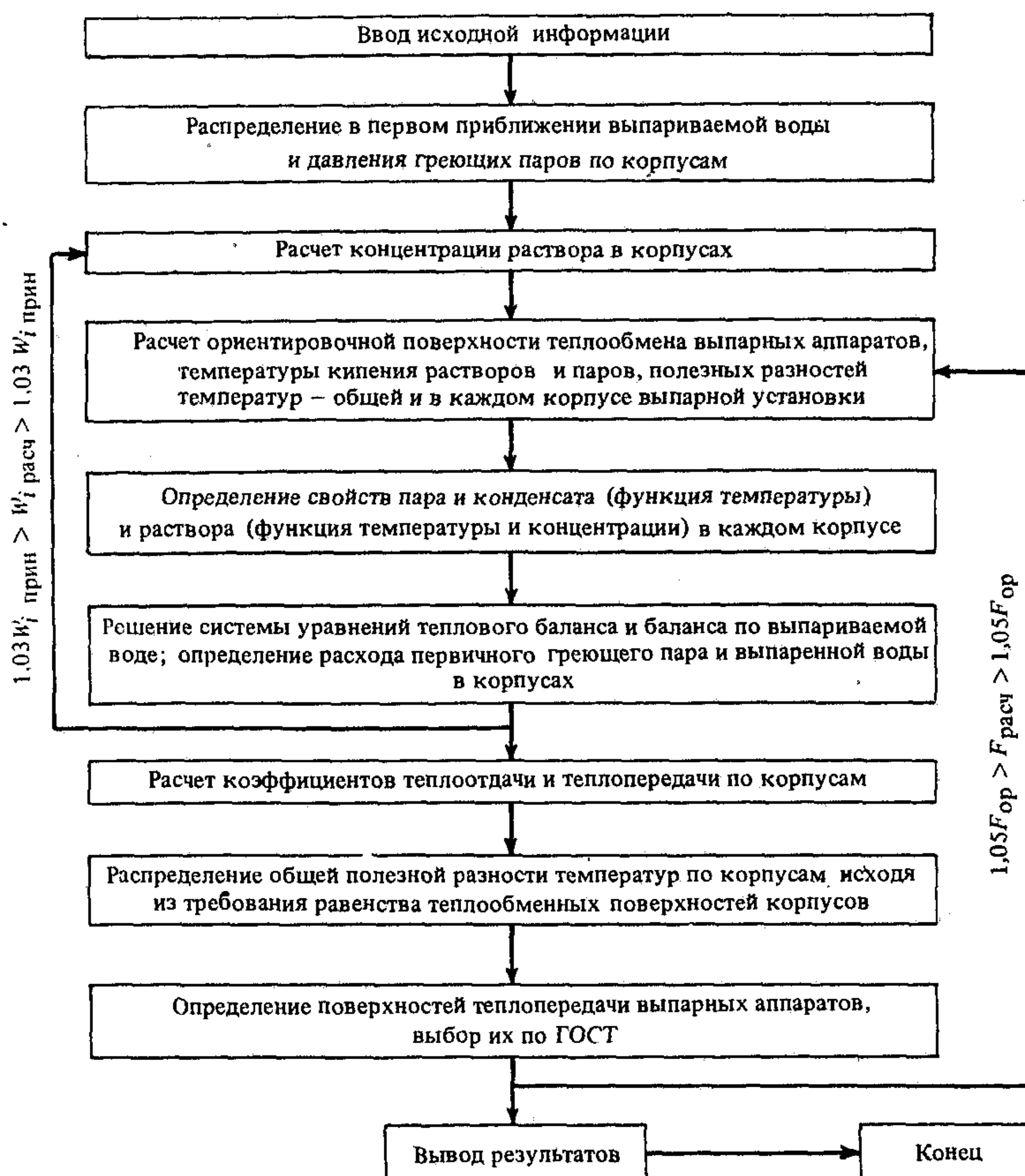
Рис. 6.11. Схема расчета многокорпусной прямоточной вакуум-выпарной установки
