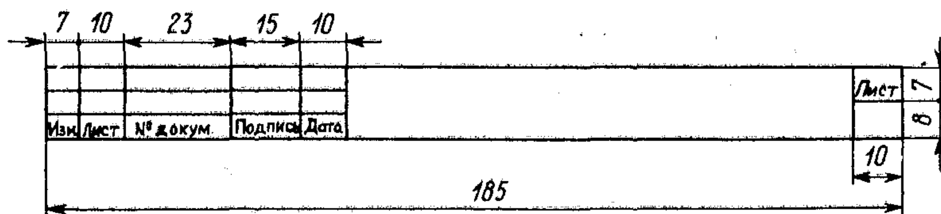
Рис. 12.5. Основная надпись для последующих листов документа
