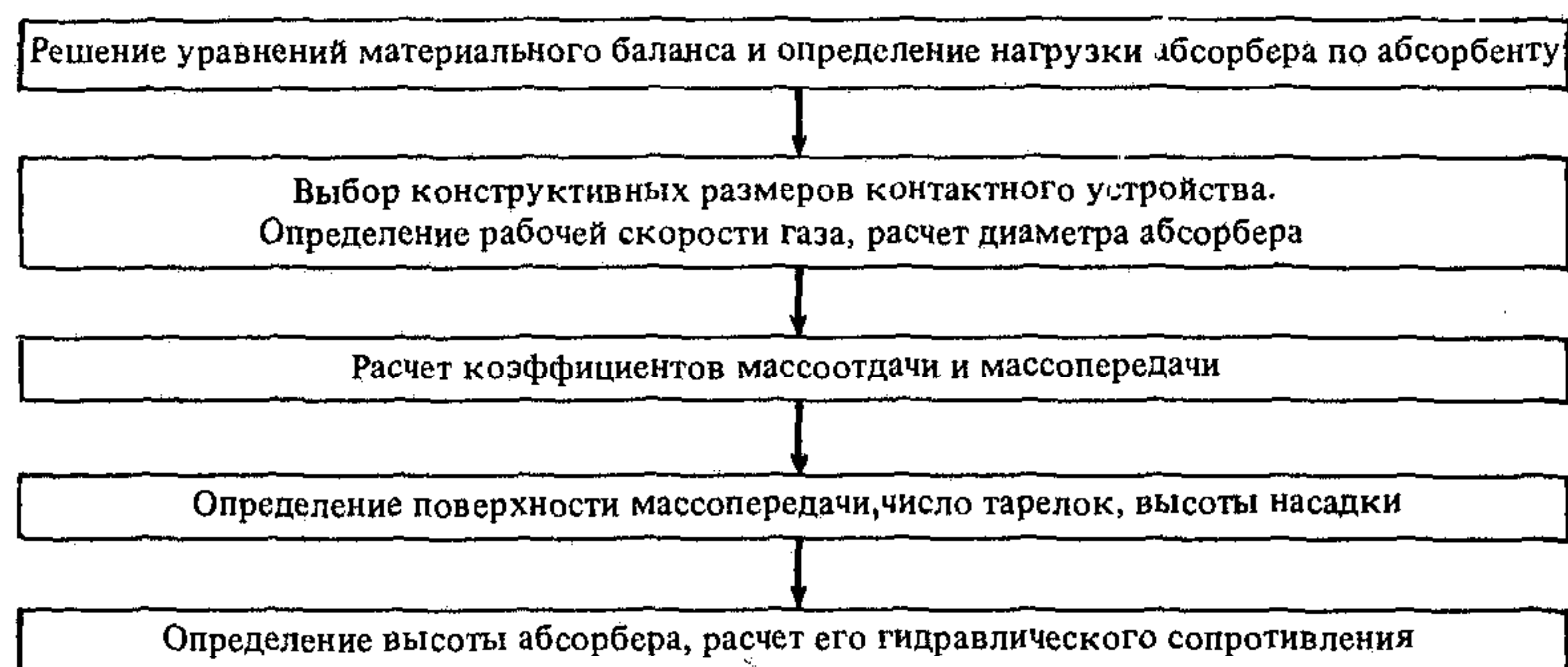
Рис. 8.1. Схема расчета абсорбционных аппаратов
