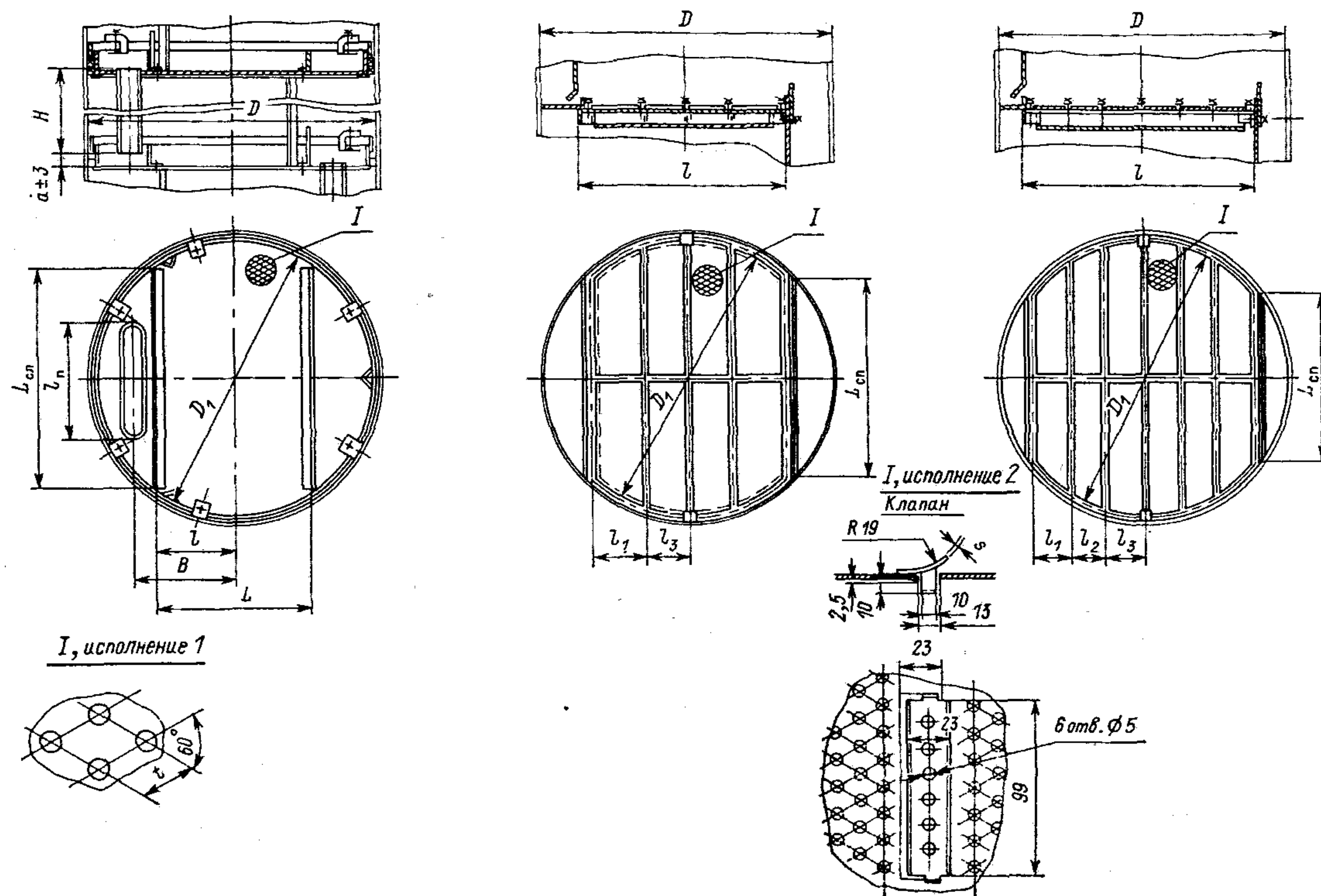
Рис. 9.13. Тарелки ситчато-клапанные колонных аппаратов: Тарелки диаметром: слева—от 400 до 800 мм; в центре—от 1000 до 2000; справа—от 2200 до 4000
