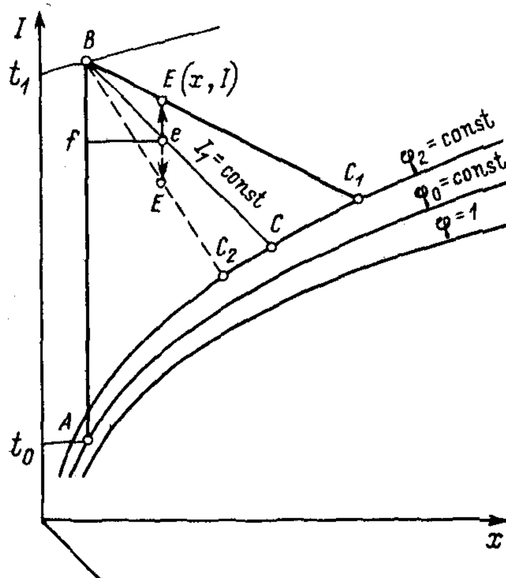
Рис. 10.1. Построение теоретического процесса сушки на I-x -диаграмме
