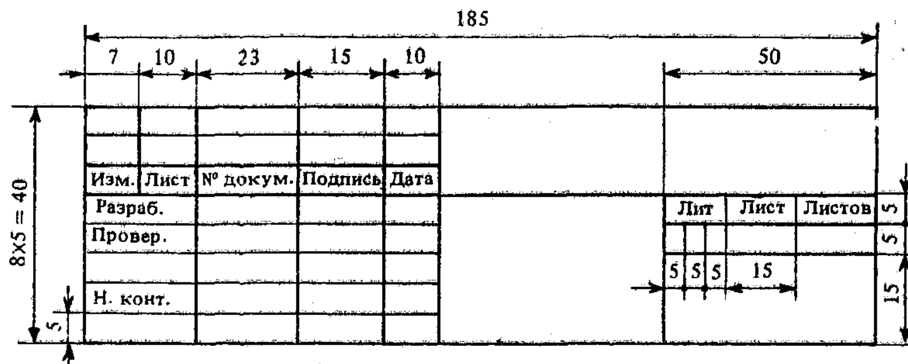
Рис. 12.4. Основная надпись для первого листа документа
