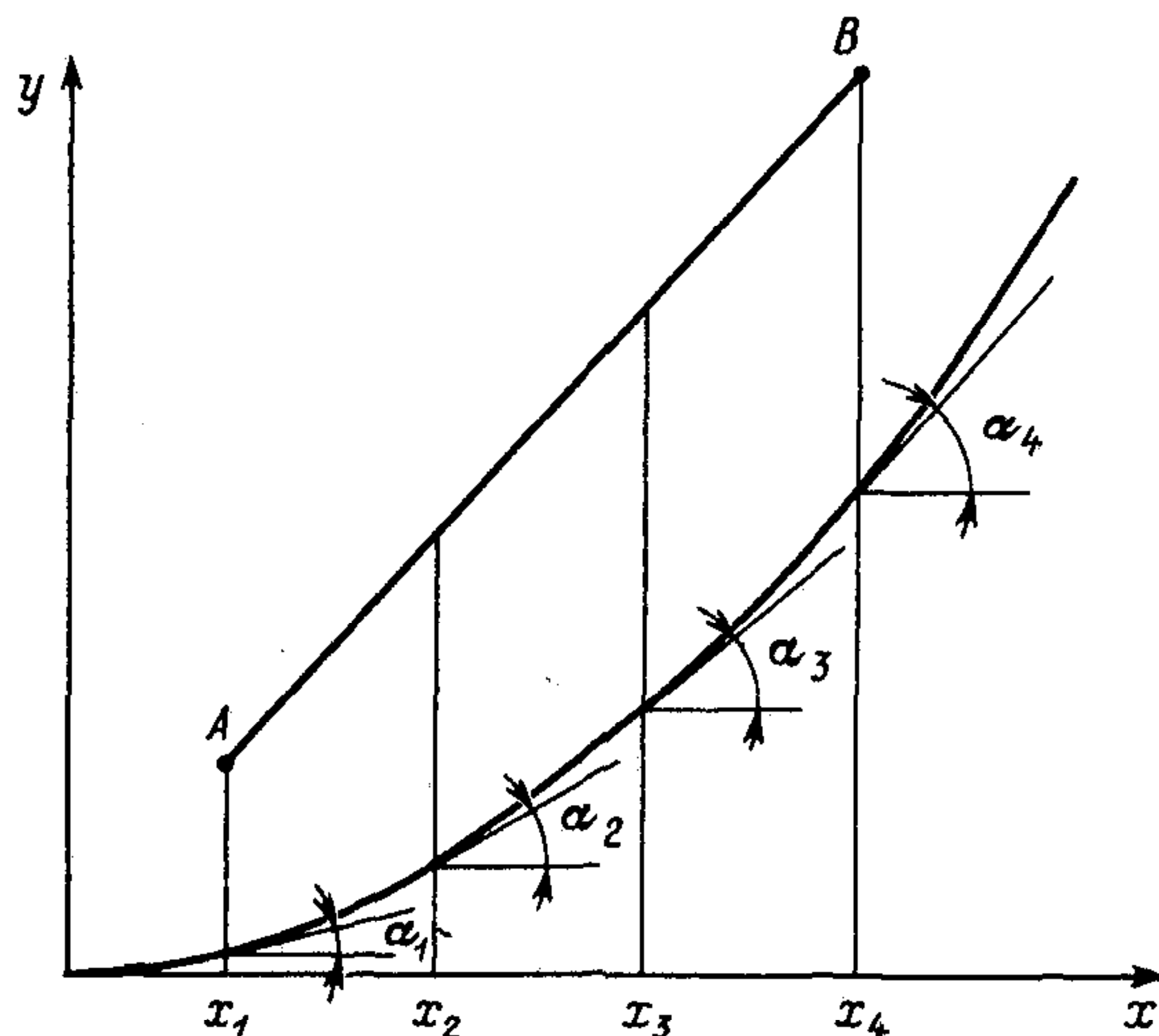
Рис. 8.10. Определение угла наклона касательных к линии равновесия
