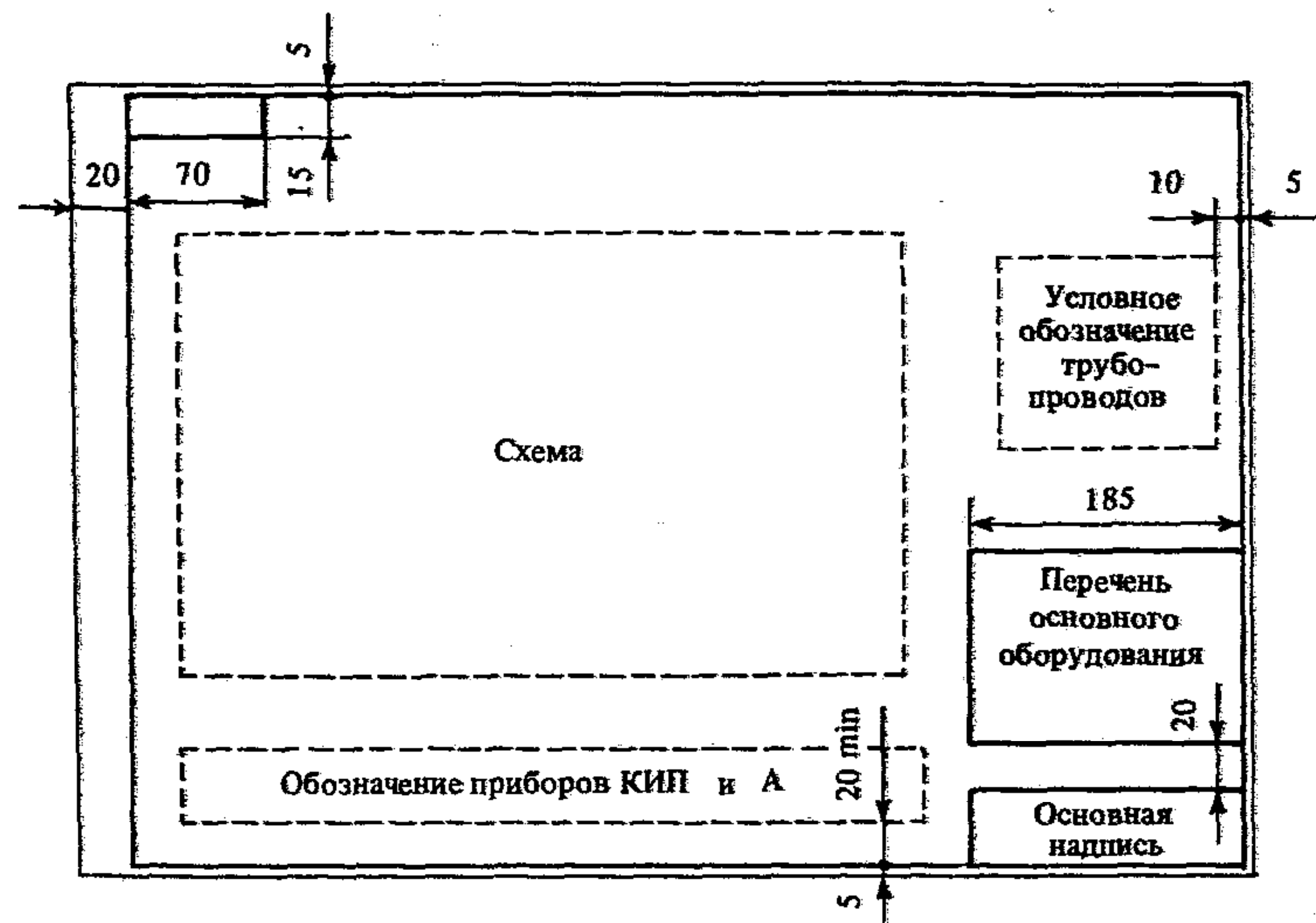
Рис. 12.7. Примерное расположение элементов чертежа технологической схемы, располагаемого короткой или длинной стороной по горизонтали
