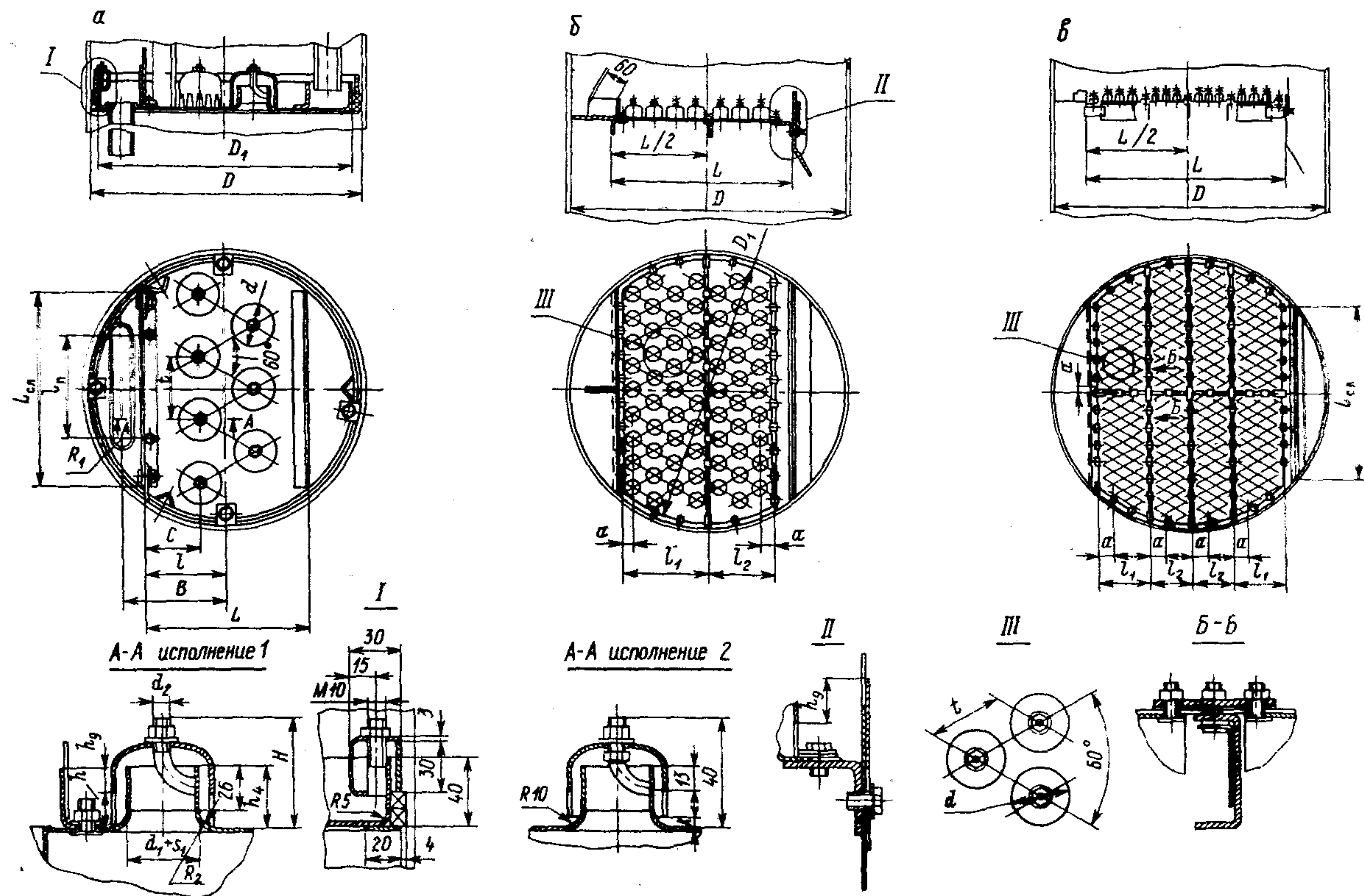
Рис. 9.12. Тарелки колпачковые стальных колонных аппаратов: Тарелки диаметром: a —от 400 до 800 мм; б —от 1000 до 2000 мм; в —от 2200 до 4000 мм
