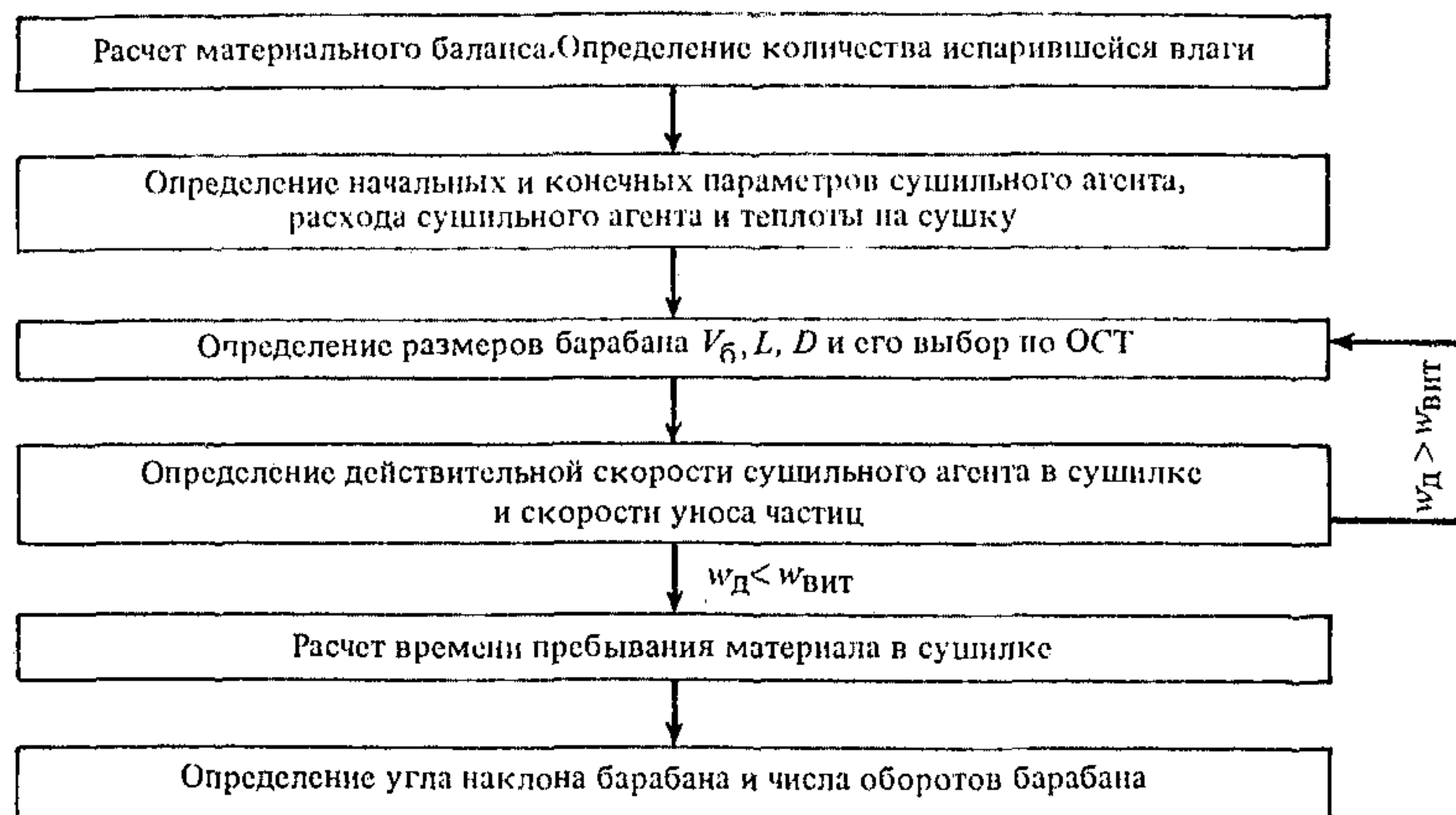
Рис. 10.4. Схема расчета барабанной сушилки, обогреваемой воздухом
