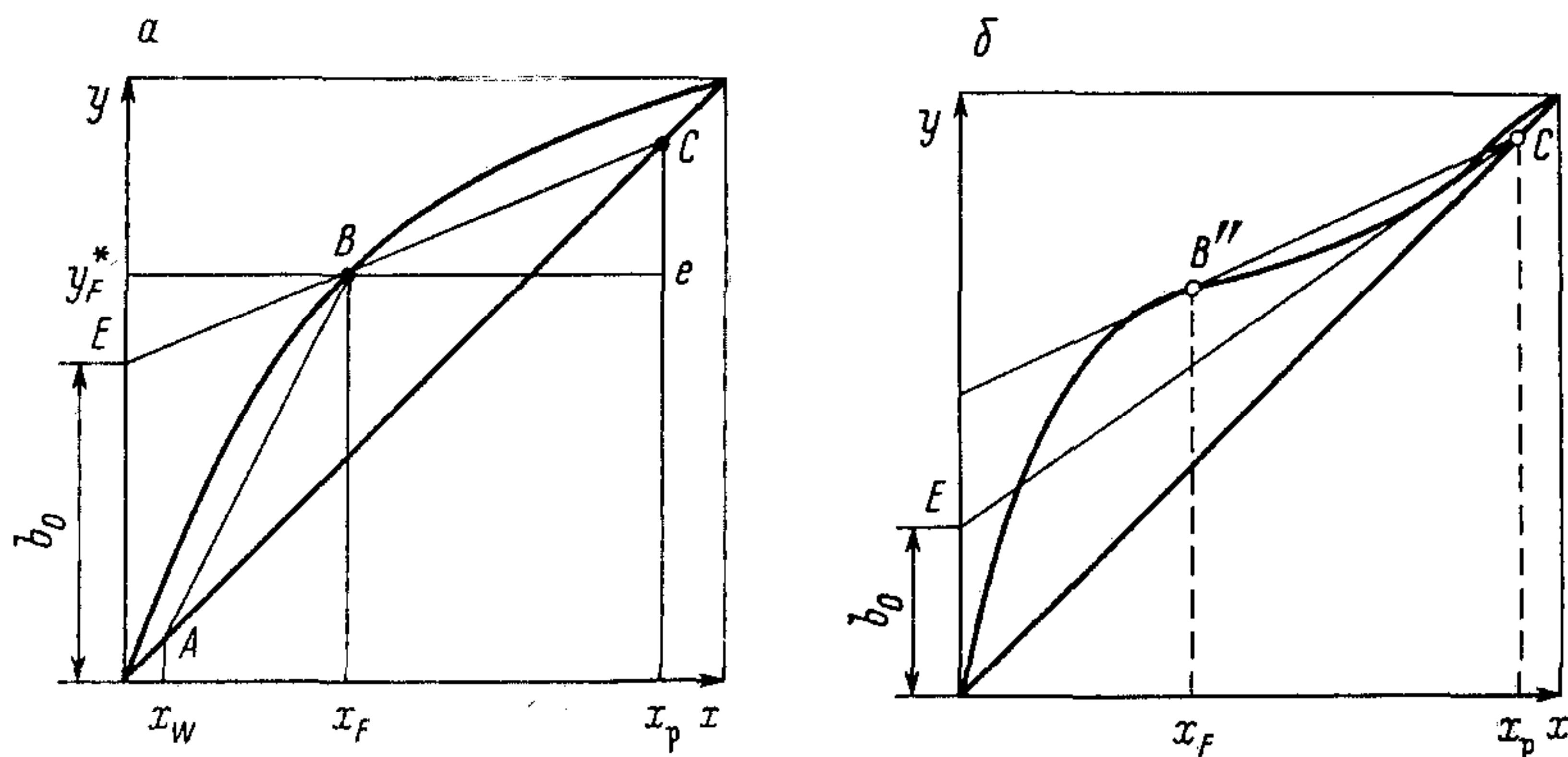
Рис. 9.1. Графическое определение минимального флегмового числа
