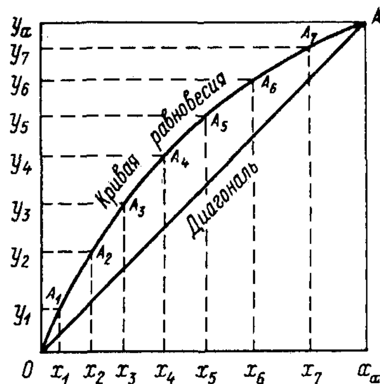
Рис. 9.3. График построения кривой равновесия
