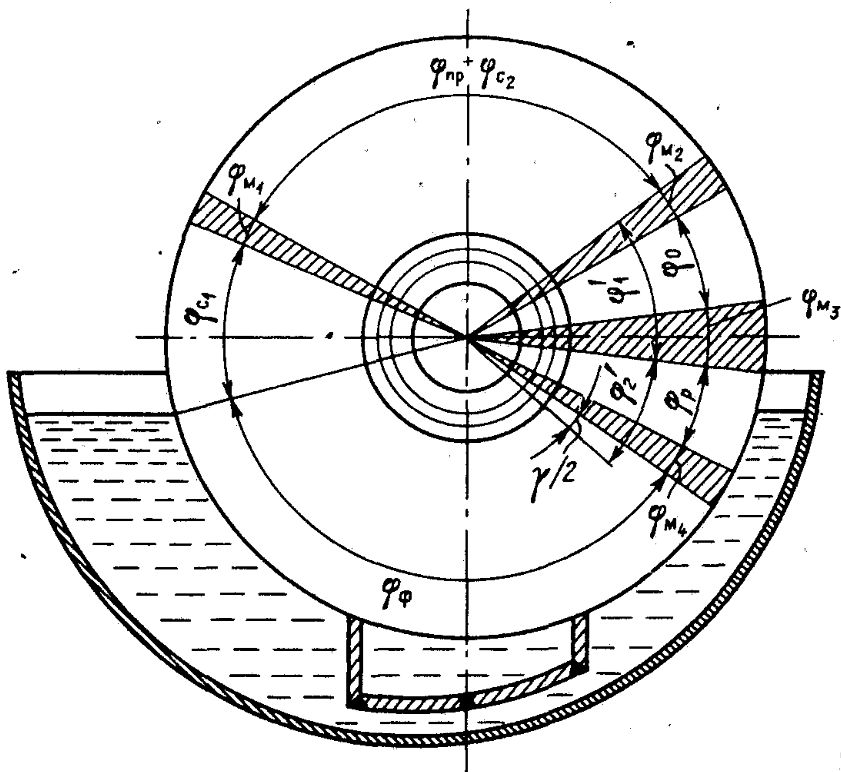
Рис. 4.6. Схема распределения технологических зон на поверхности барабана
