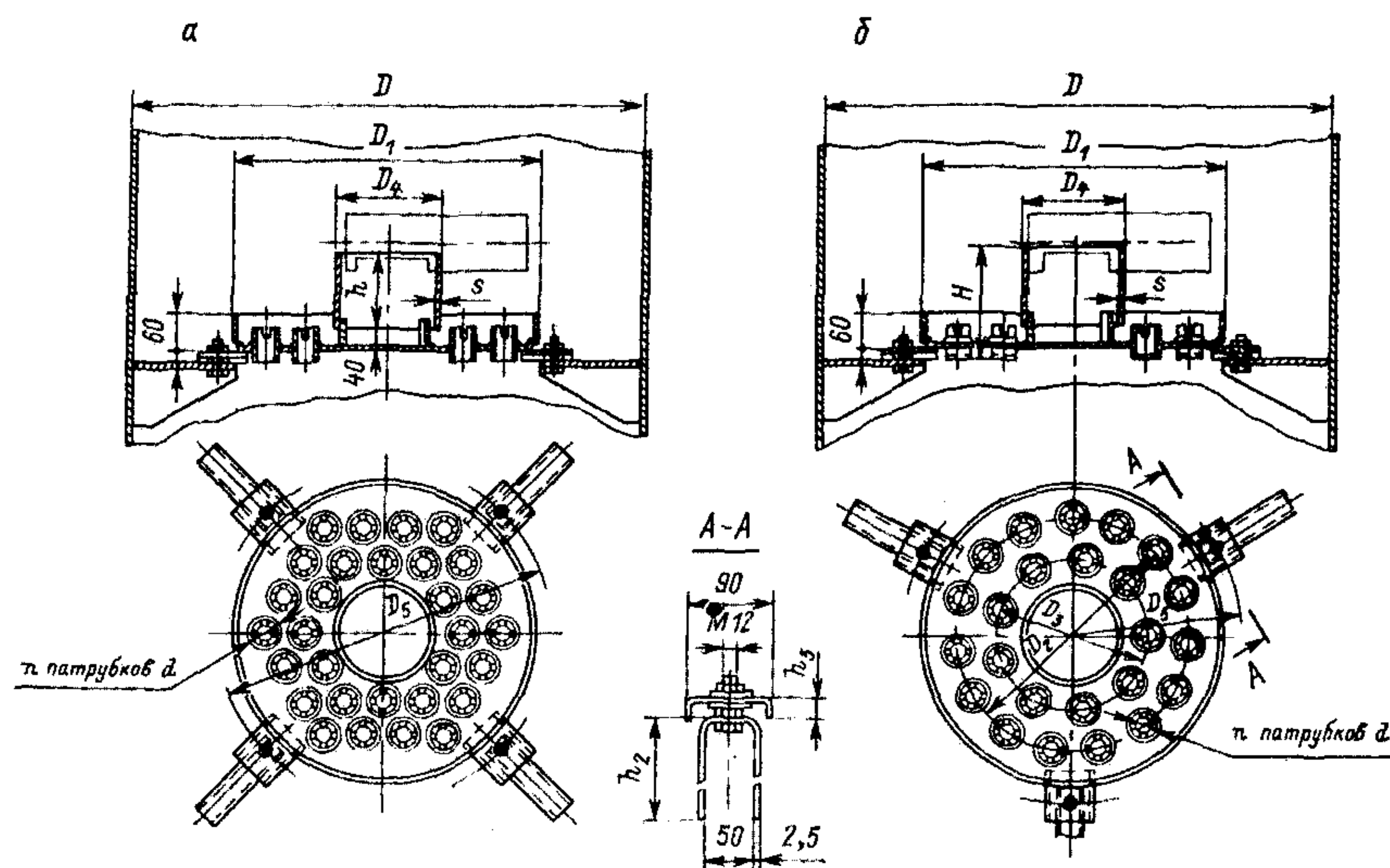
Рис. 8.16. Тарелка ТСН-3:
