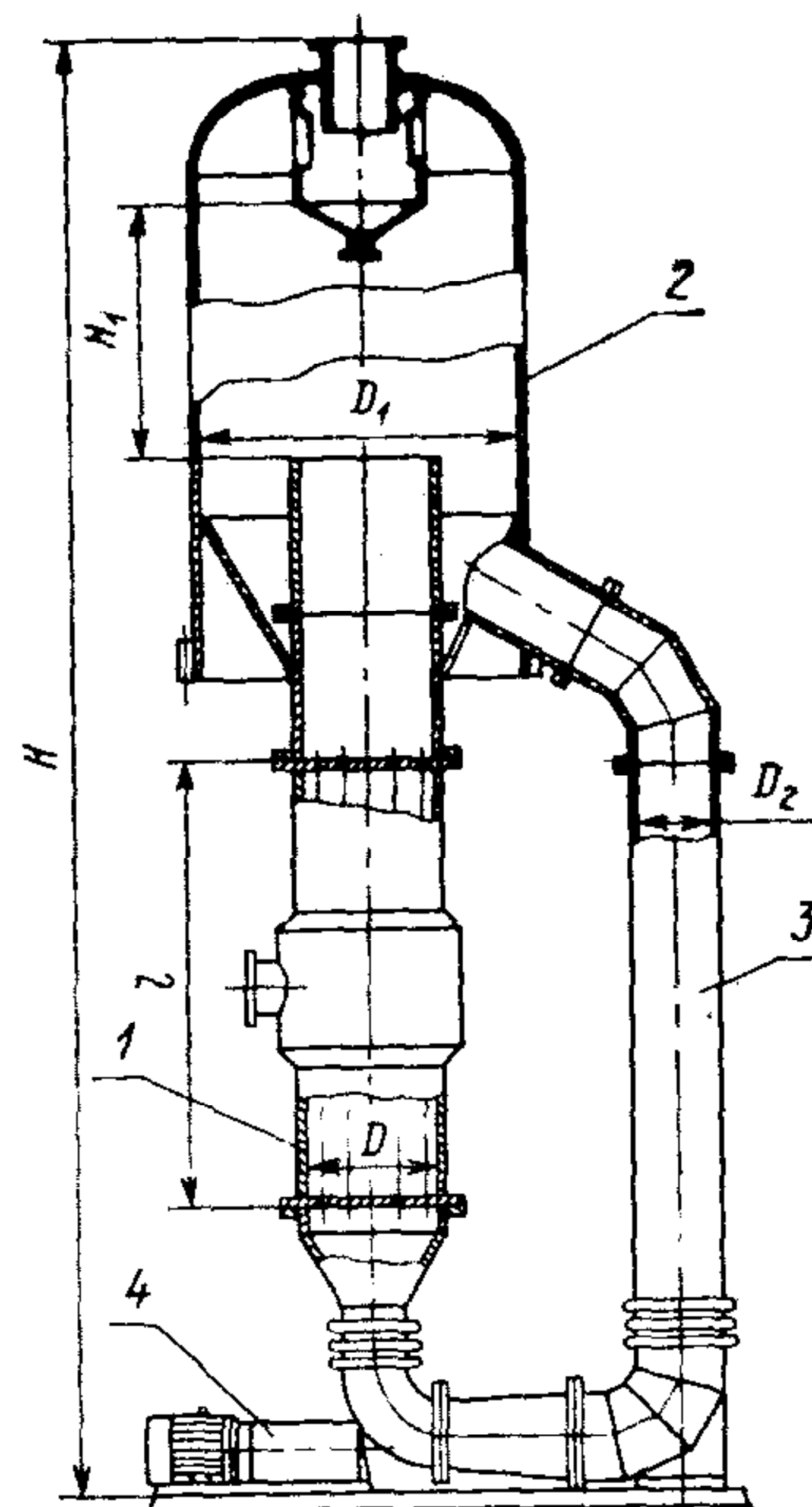
Рис. 6.16. Выпарной аппарат (тип 2, исполнение 2): 1—греющая камера; 2—сепаратор; 3—циркуляционная труба; 4—элек- тронасосный агрегат
