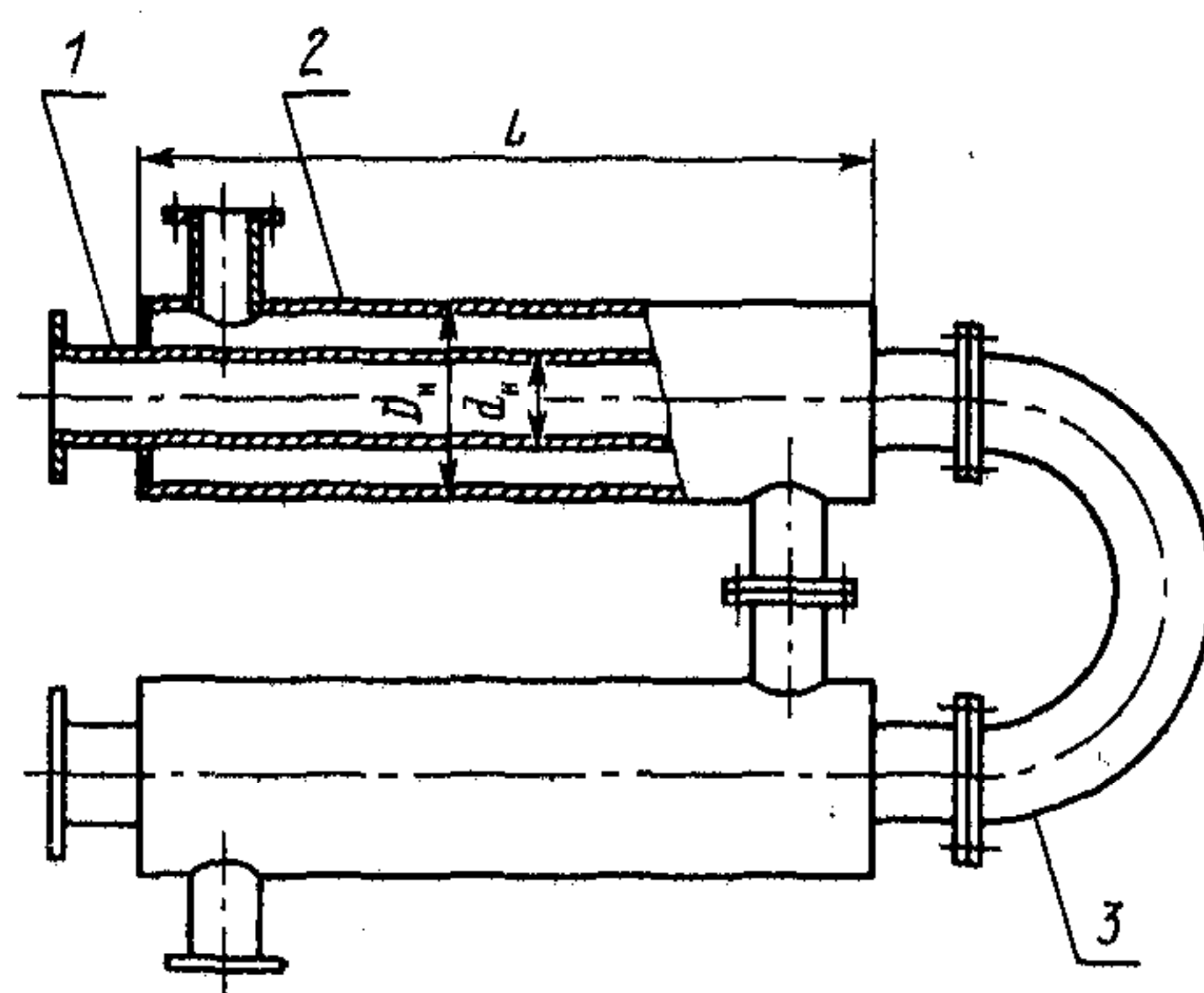
Рис. 5.10. Теплообменник типа «труба в трубе»:
