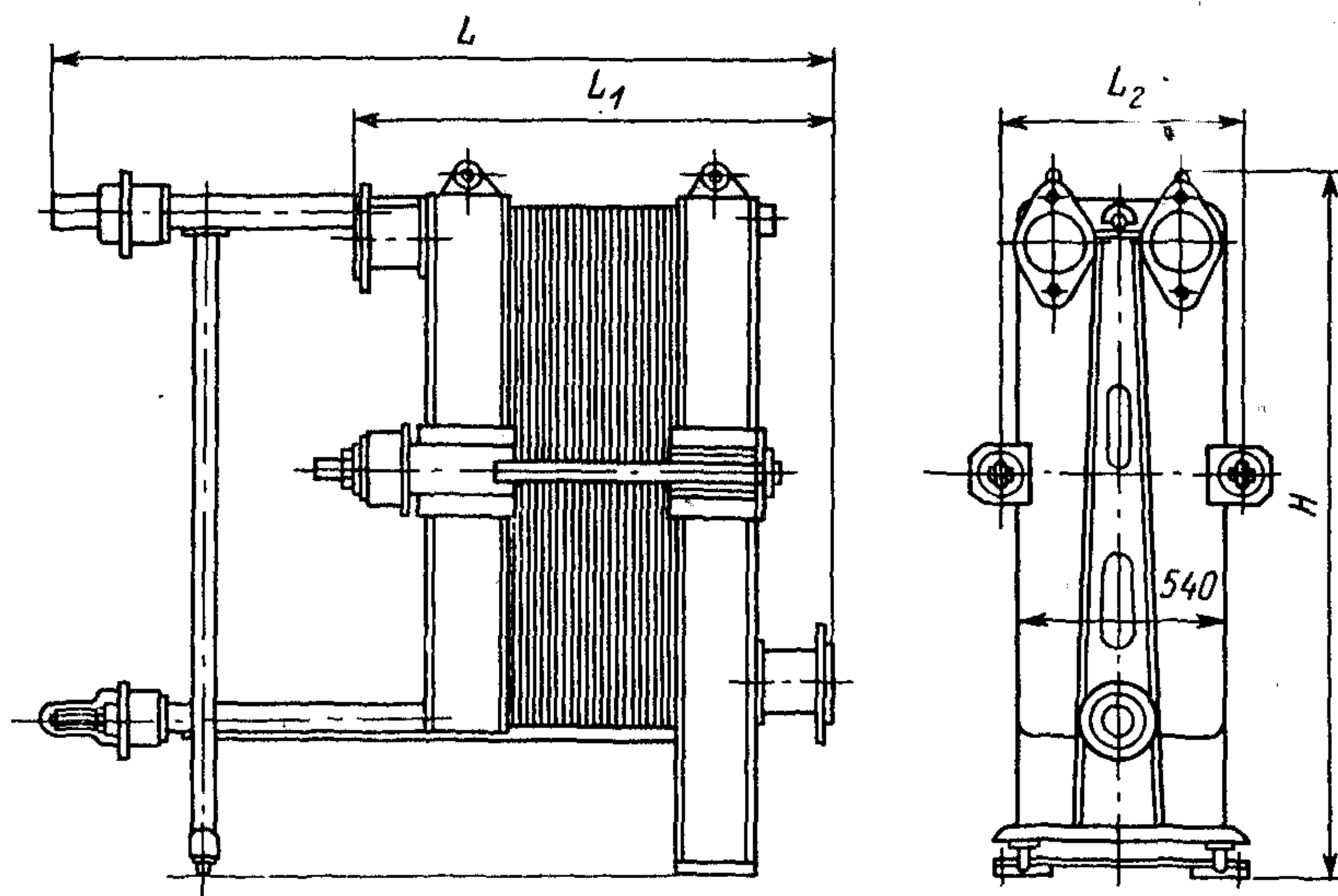
Рис. 5.13. Пластинчатый теплообменник на двухопорной раме
