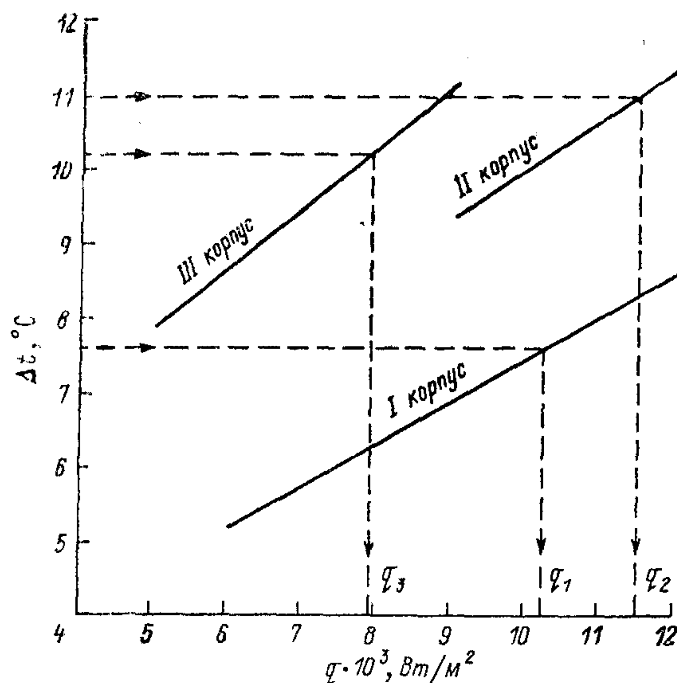
Рис. 6.10. Определение тепловых нагрузок выпарных аппаратов
