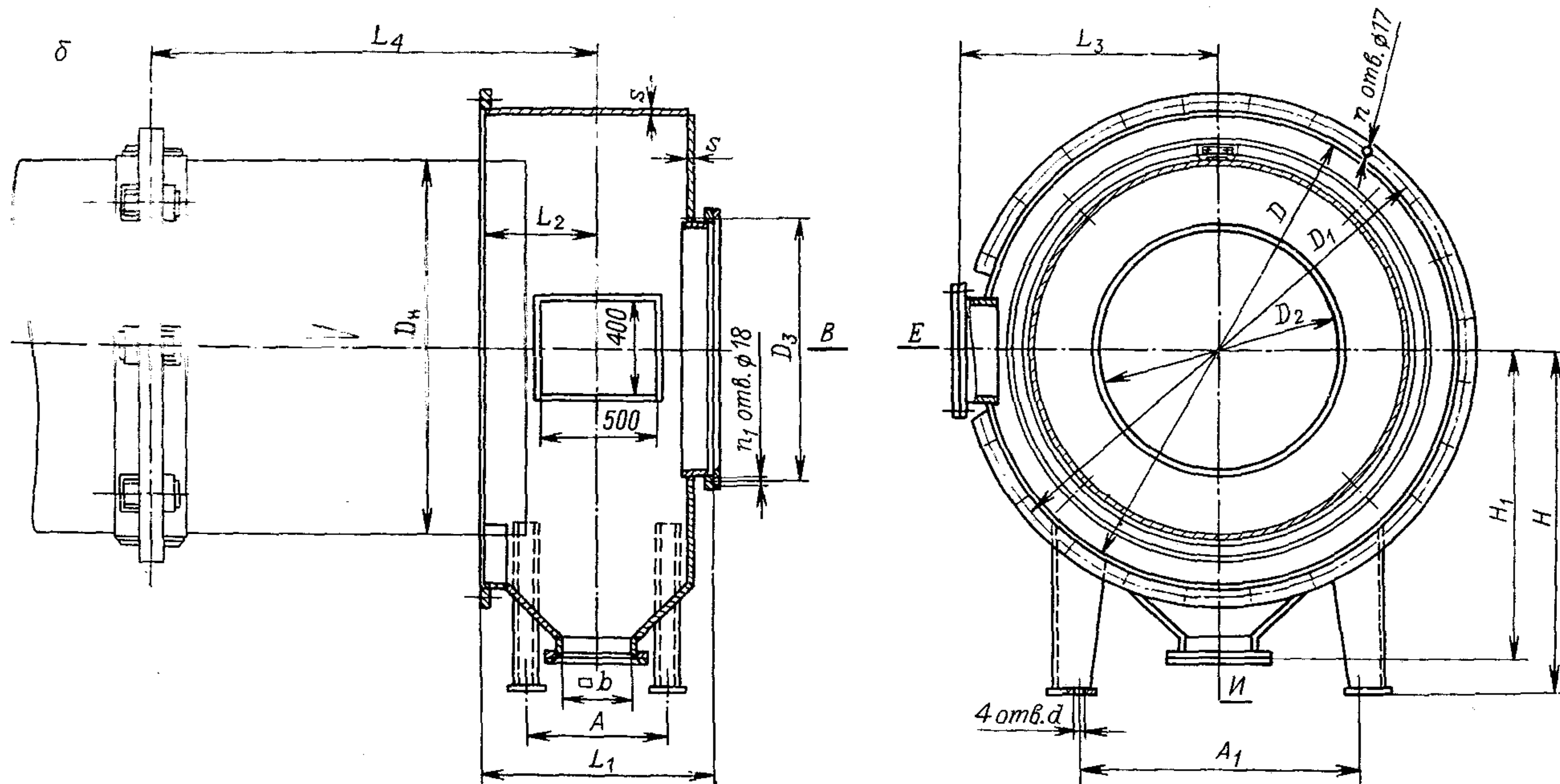
Рис. 10.12. Загрузочная (а) и разгрузочная (б) камеры для сушилок с противоточным движением потоков
