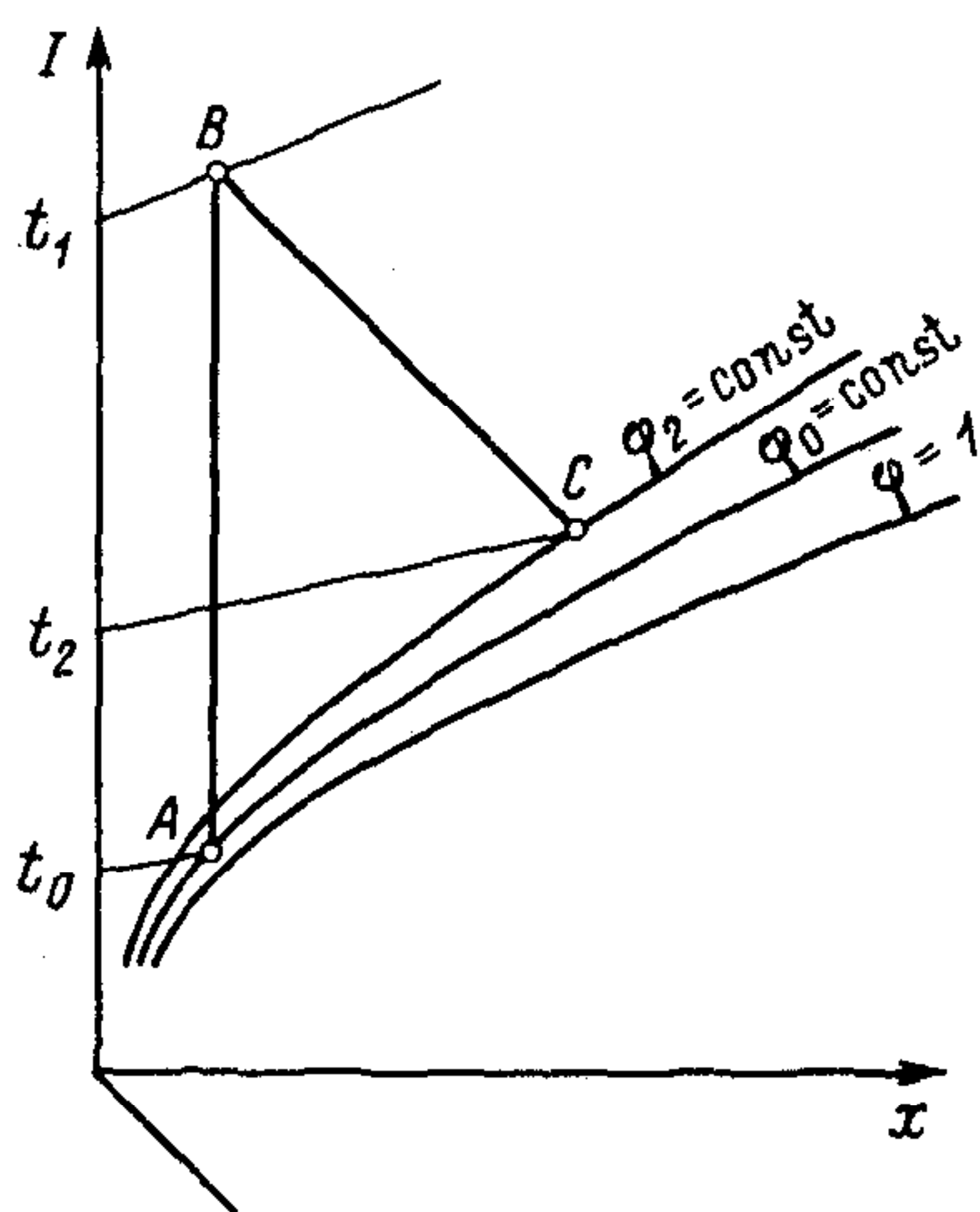
Рис. 10.1. Построение теоретического процесса сушки на I-x -диаграмме
