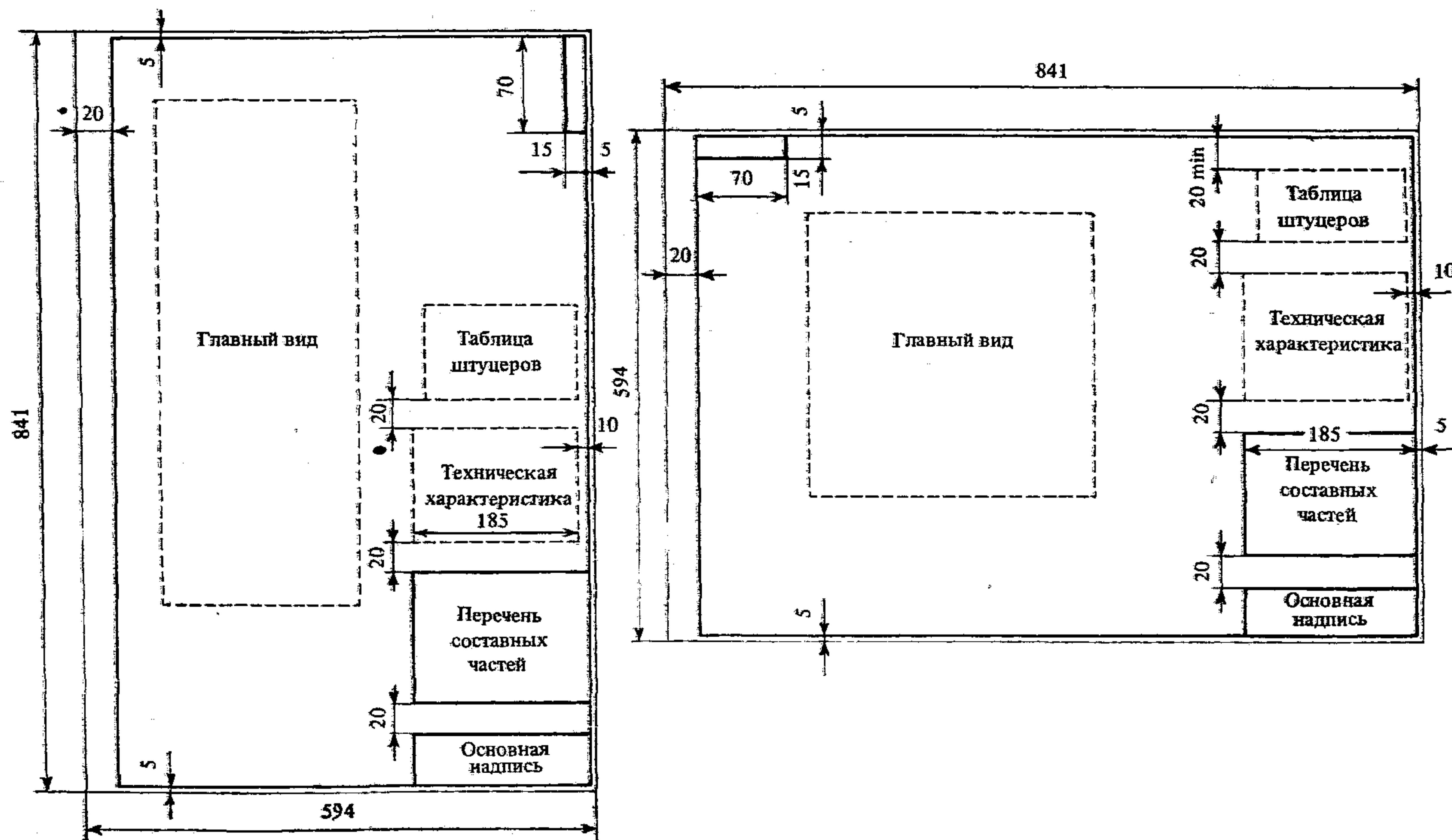
Рис. 12.11. Примерное расположение элементов чертежа общего вида, располагаемого короткой или длинной стороной по горизонтали
