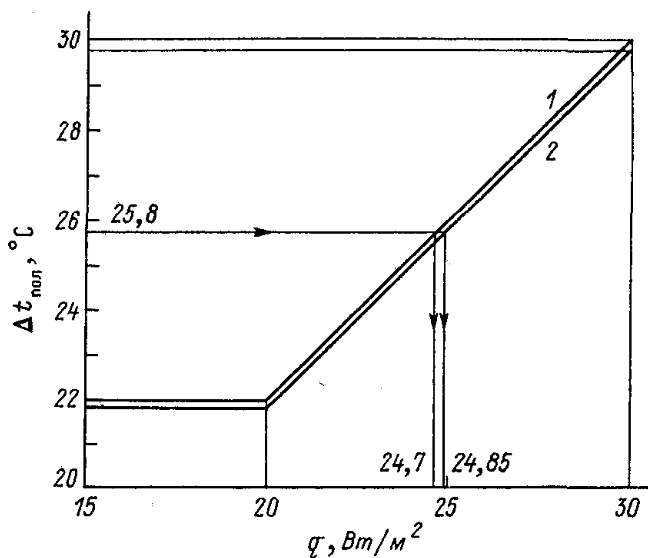
Рис. 6.7. Определение удельной тепловой нагрузки выпарного аппарата
