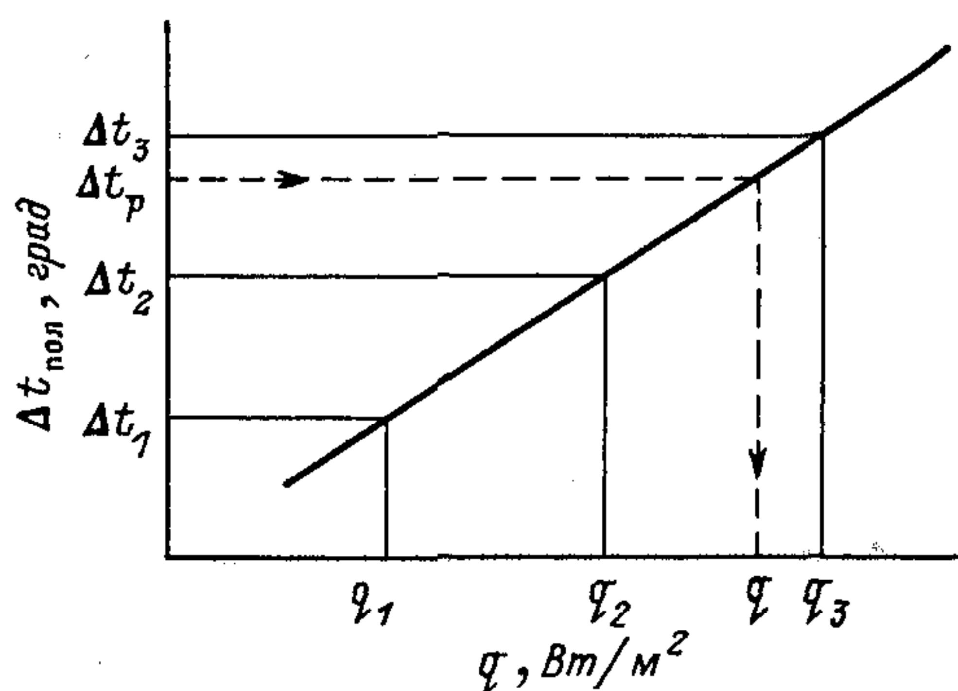
Рис. 6.2. Определение удельной тепловой нагрузки q выпарного аппарата
