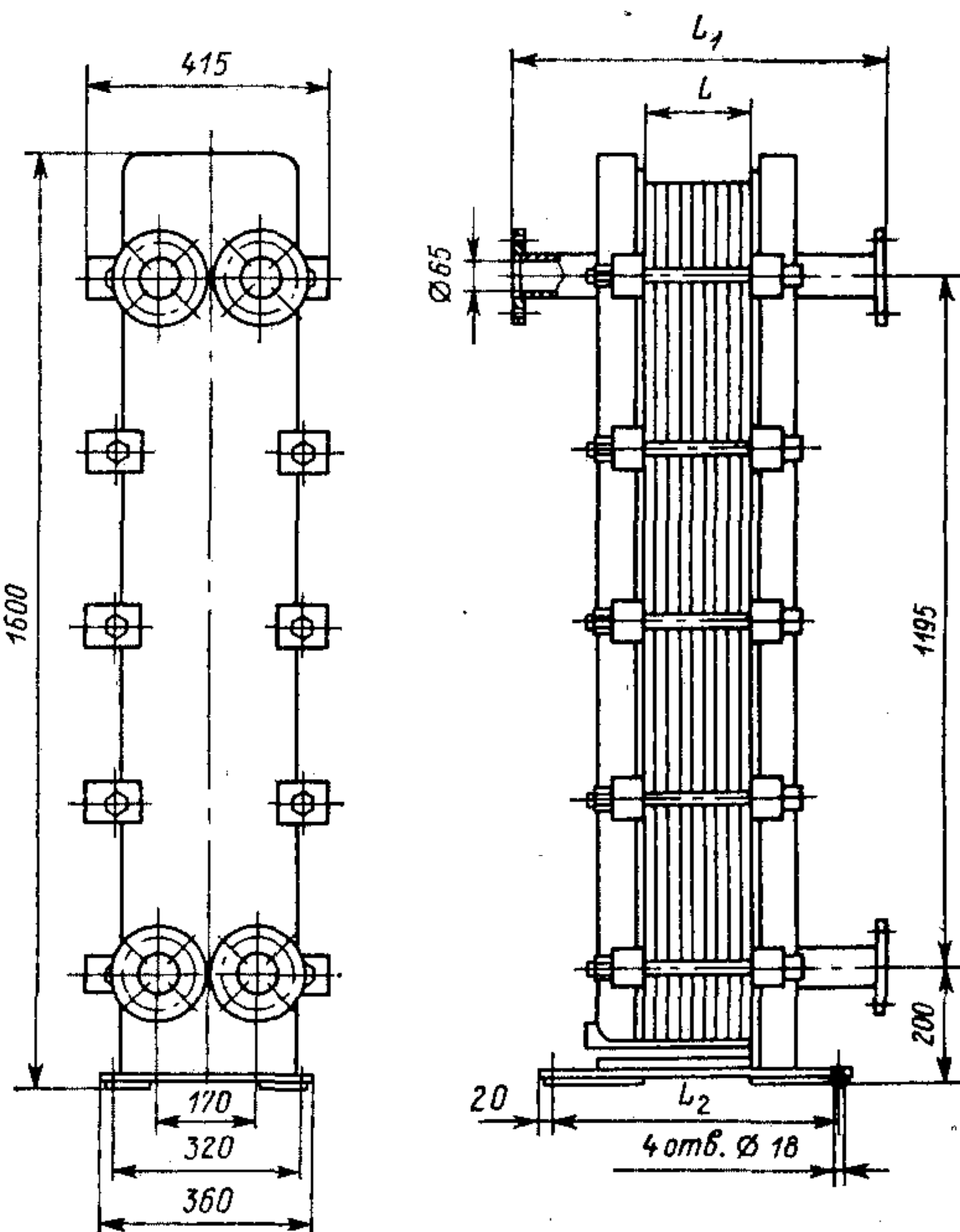
Рис. 5.12. Пластинчатый теплообменник на консольной раме
