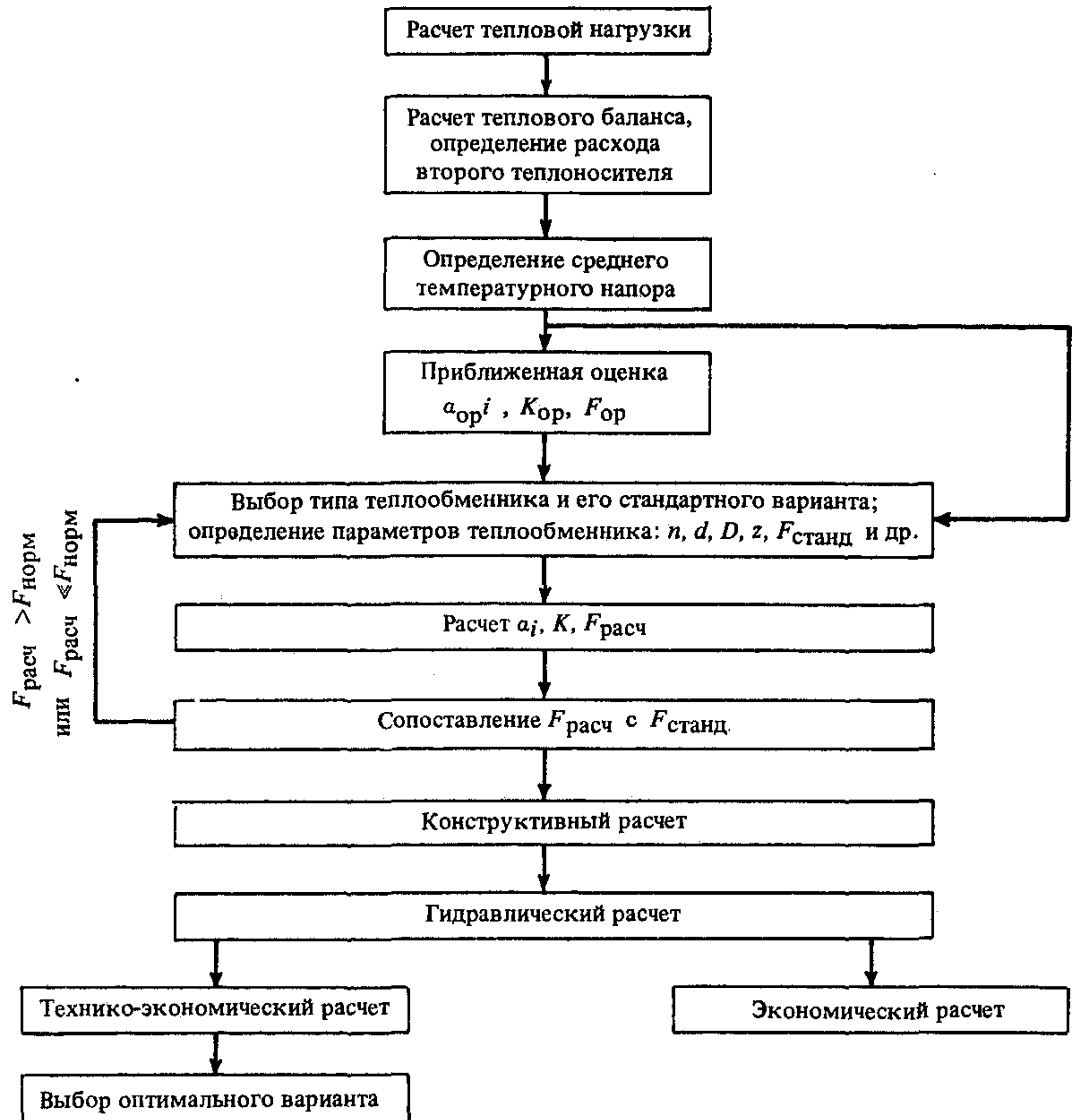
Рис. 5.1. Схема расчета теплообменников
