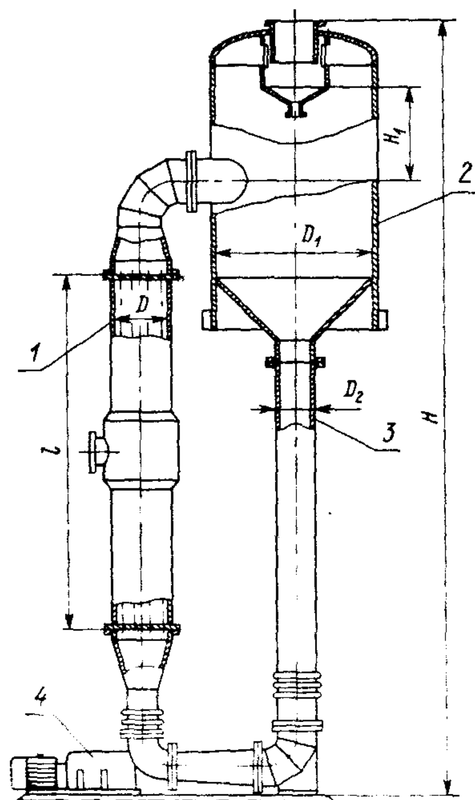
Рис. 6.15. Выпарной аппарат (тип 2, исполнение 1): 1—греющая камера; 2—сепаратор; 3—циркуляционная труба; 4—электро- насосный агрегат
