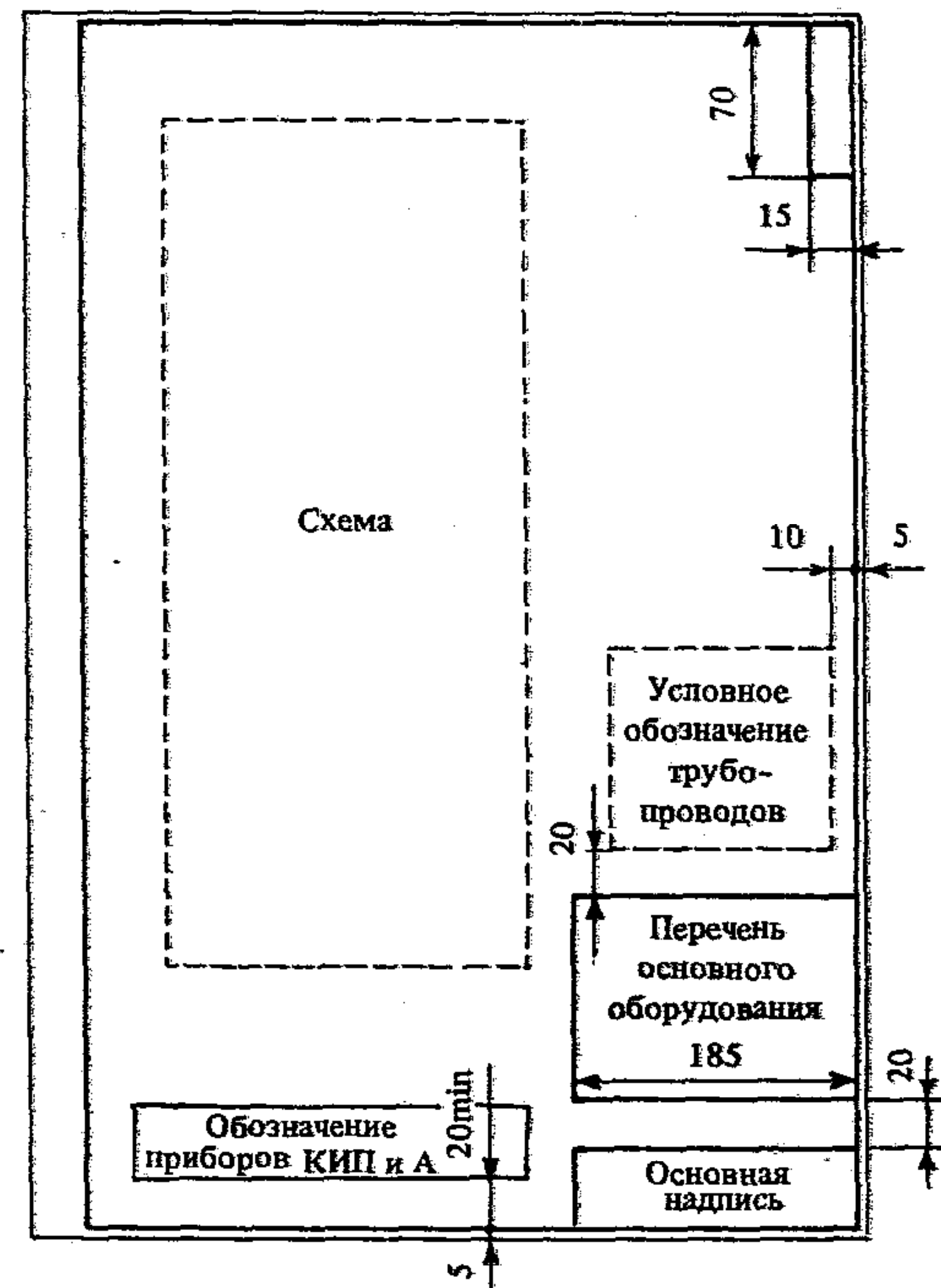
Рис. 12.7. Примерное расположение элементов чертежа технологической схемы, располагаемого короткой или длинной стороной по горизонтали
