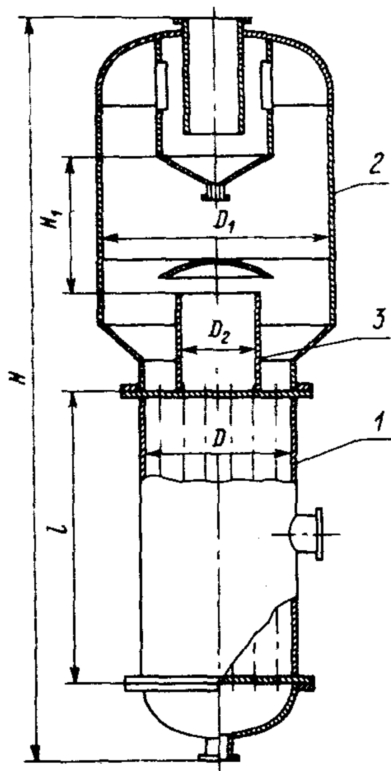
Рис. 6.12. Выпарной аппарат (тип 1, исполнение 1): 1—греющая камера; 2—сепаратор; 3—распределительная камера
