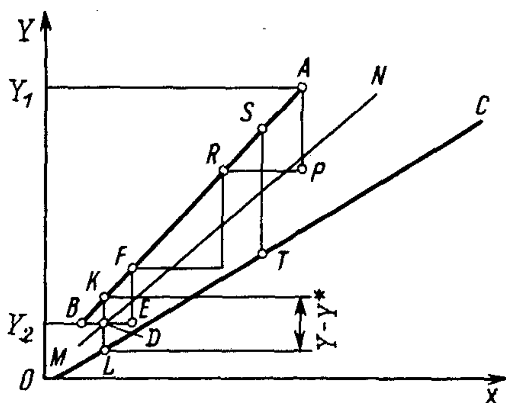
Рис. 8.6. Графическое определение числа единиц переноса
