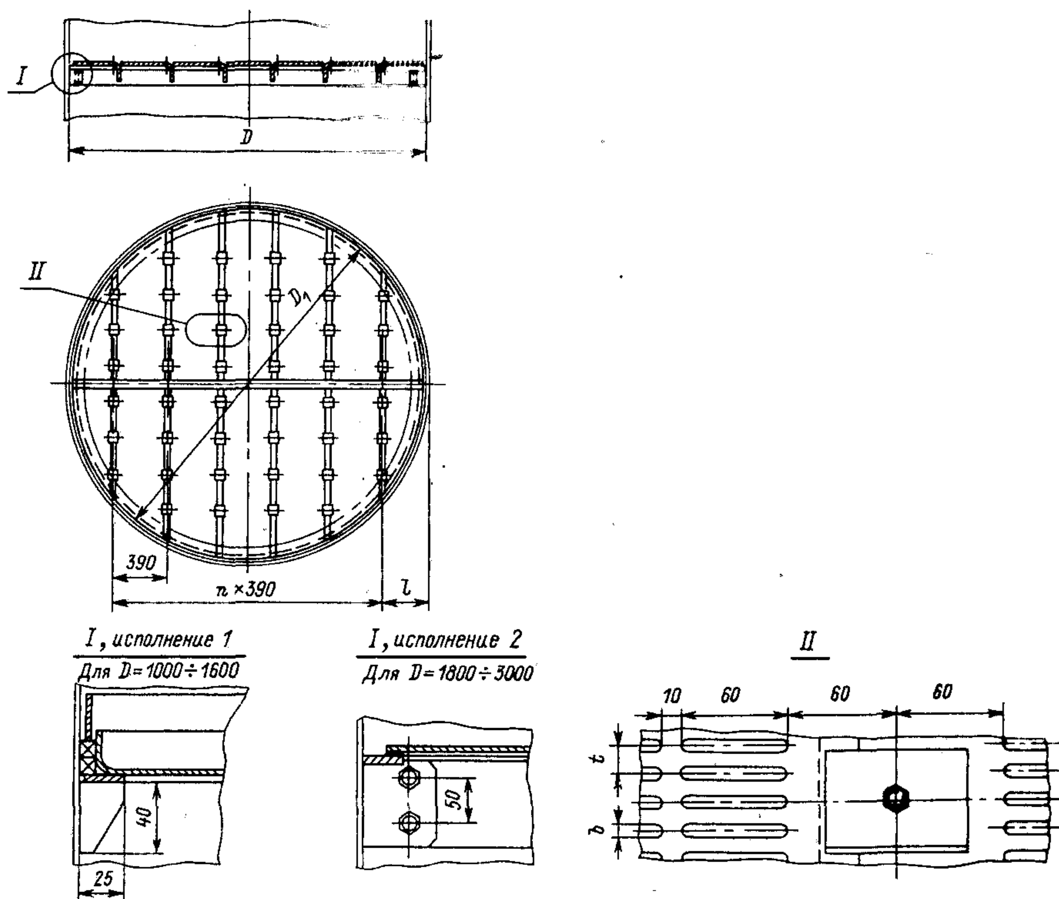
Рис. 9.14. Тарелки решетчатые провального типа
