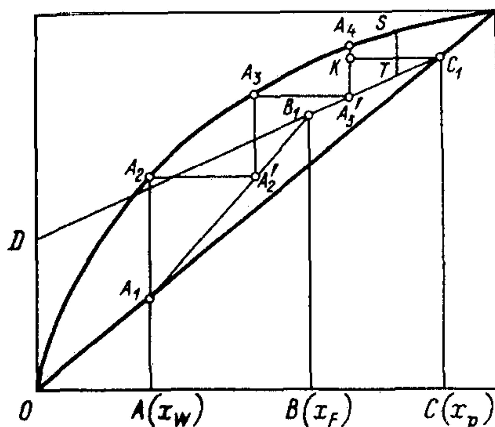
Рис. 9.5. Построение линий рабочих концентраций укрепляющей и истощающей части колонны
