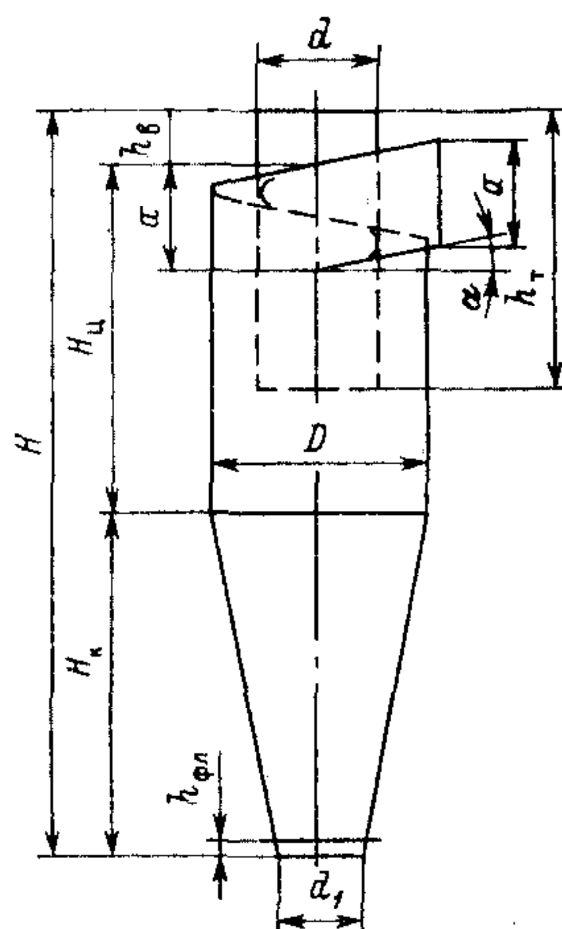
Рис. 10.5. Циклон типа ЦН
