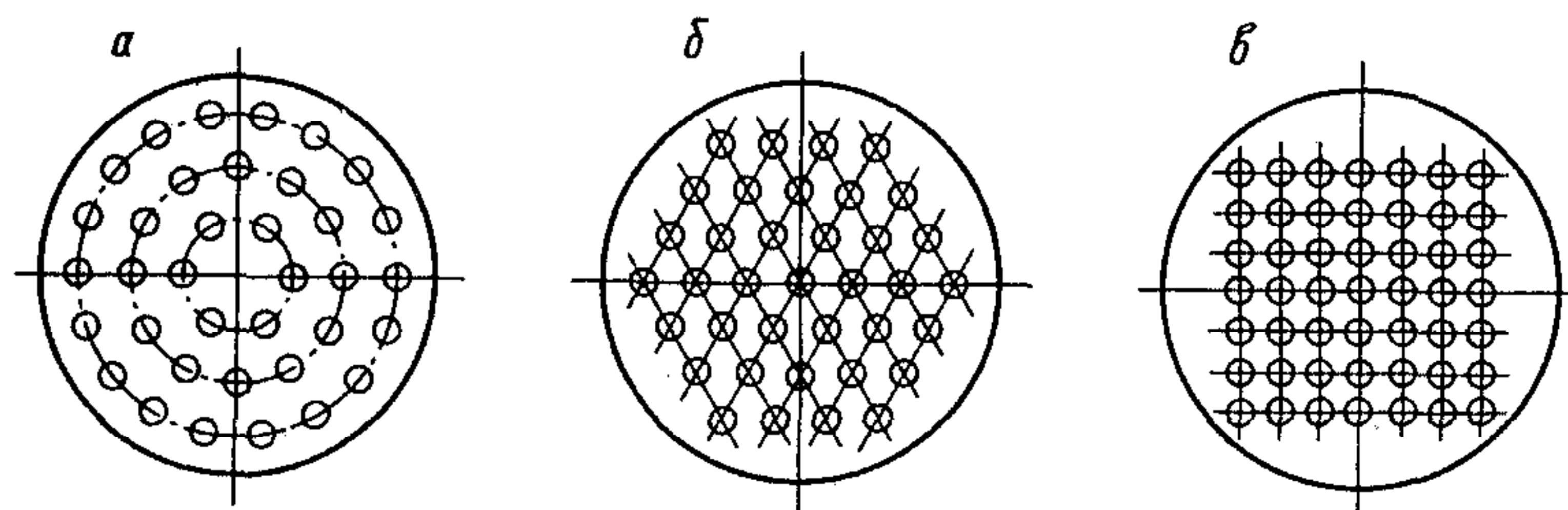
Рис. 5.4. Размещение труб в трубных решетках теплообменников:
