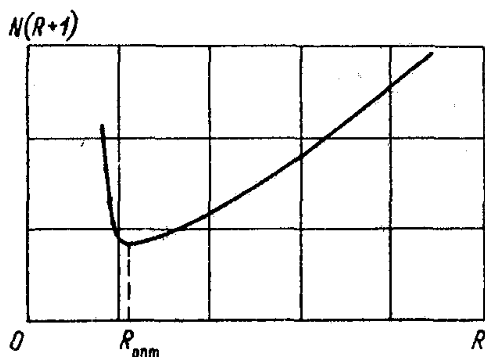
Рис. 9.2. Определение оптимального рабочего флегмового числа
