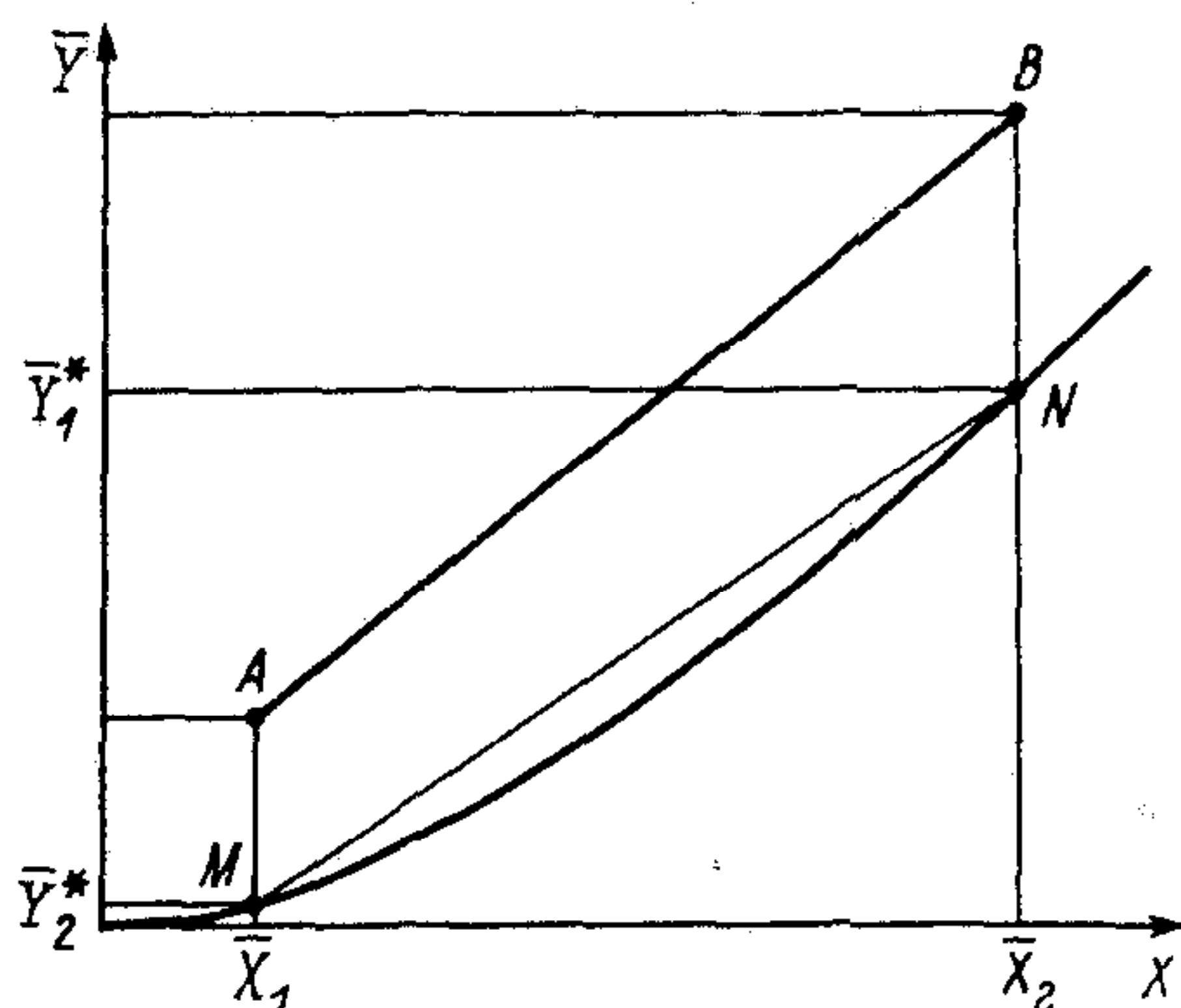
Рис. 8.7. Определение угла наклона линии равновесия
