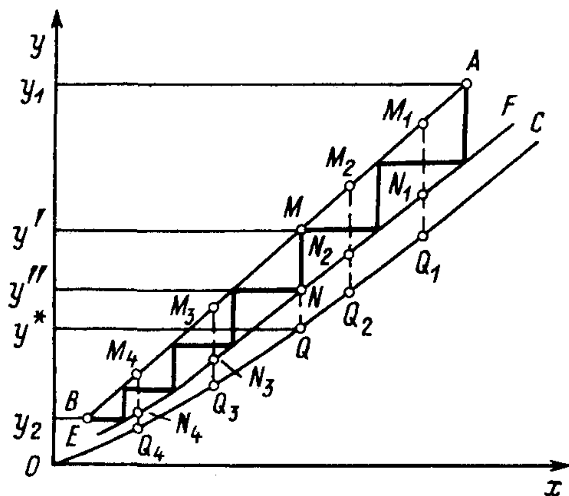
ответствующей составу газа и жидкости на входе в аппарат, вписывают между рабочей и кинетической кривой ступенчатую линию из вертикальных и горизонтальных участков отрезков, как показано на рис. 8.9. Число вертикальных отрезков этой ступенчатой линии между начальным и
