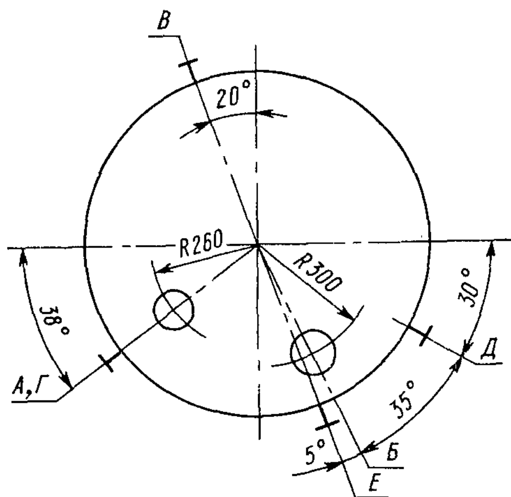
Рис. 12.9. Схема расположения штуцеров бобышек, люков
