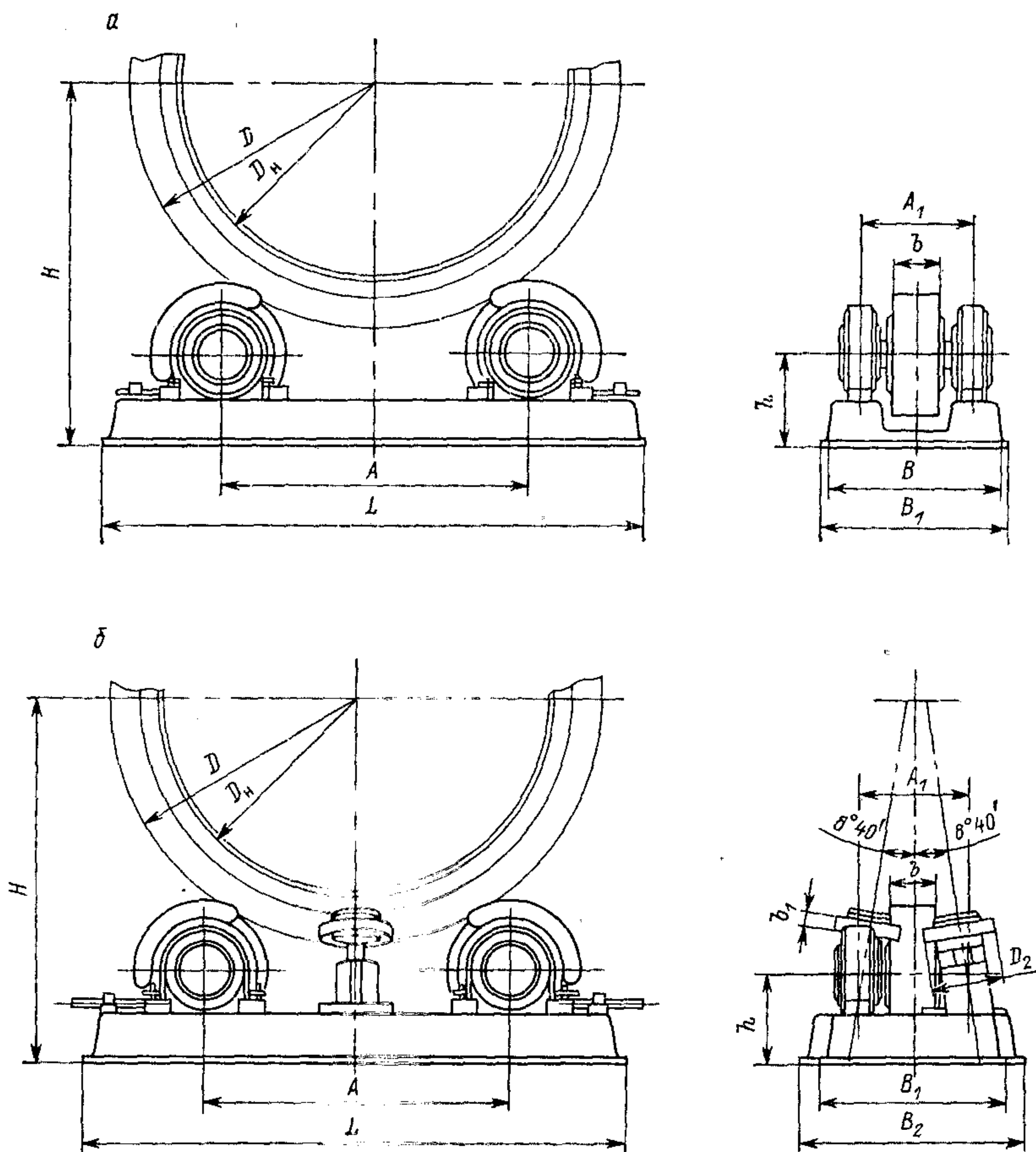
Рис. 10.10. Станции опорная (а) и упорно-опорная (б)
