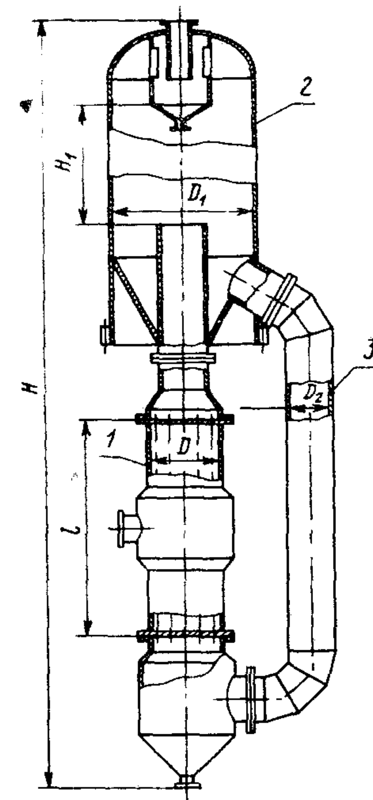
Рис. 6.14. Выпарной аппарат (тип 1, исполнение 3): 1—греющая камера; 2—сепаратор; 3—циркуляционная труба
