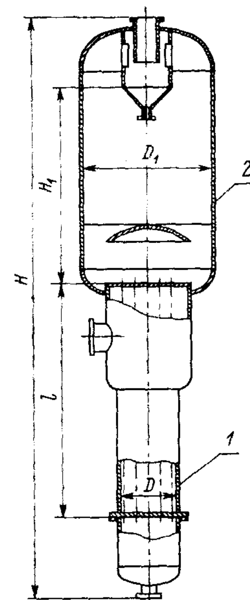
Рис. 6.17. Выпарной аппарат (тип 3, исполнение 1): 1—греющая камера; 2—сепаратор
