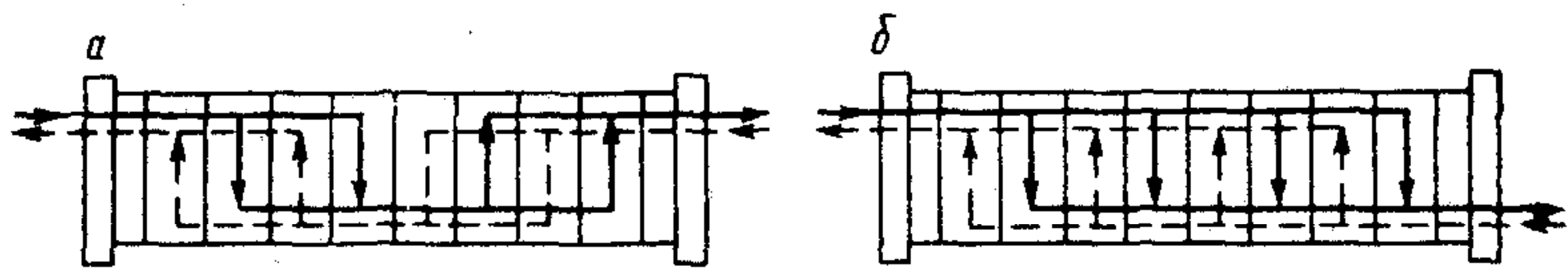
Рис. 5.8. Примеры компоновки пластин;
