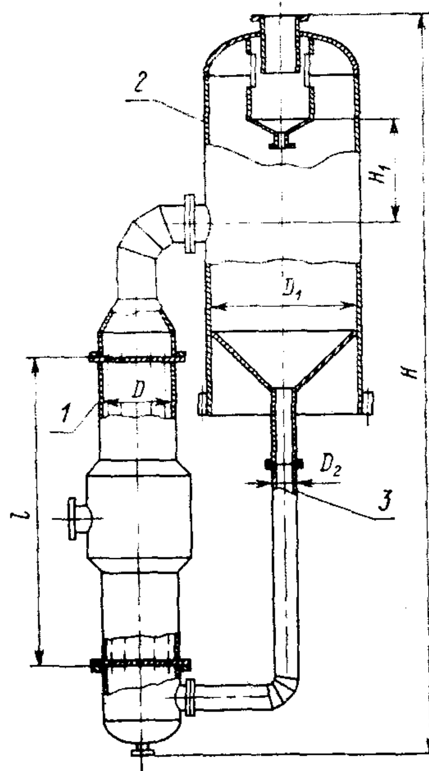
Рис. 6.13. Выпарной аппарат (тип 1, исполнение 2): 1—греющая камера; 2—сепаратор; 3—циркуляционная труба
