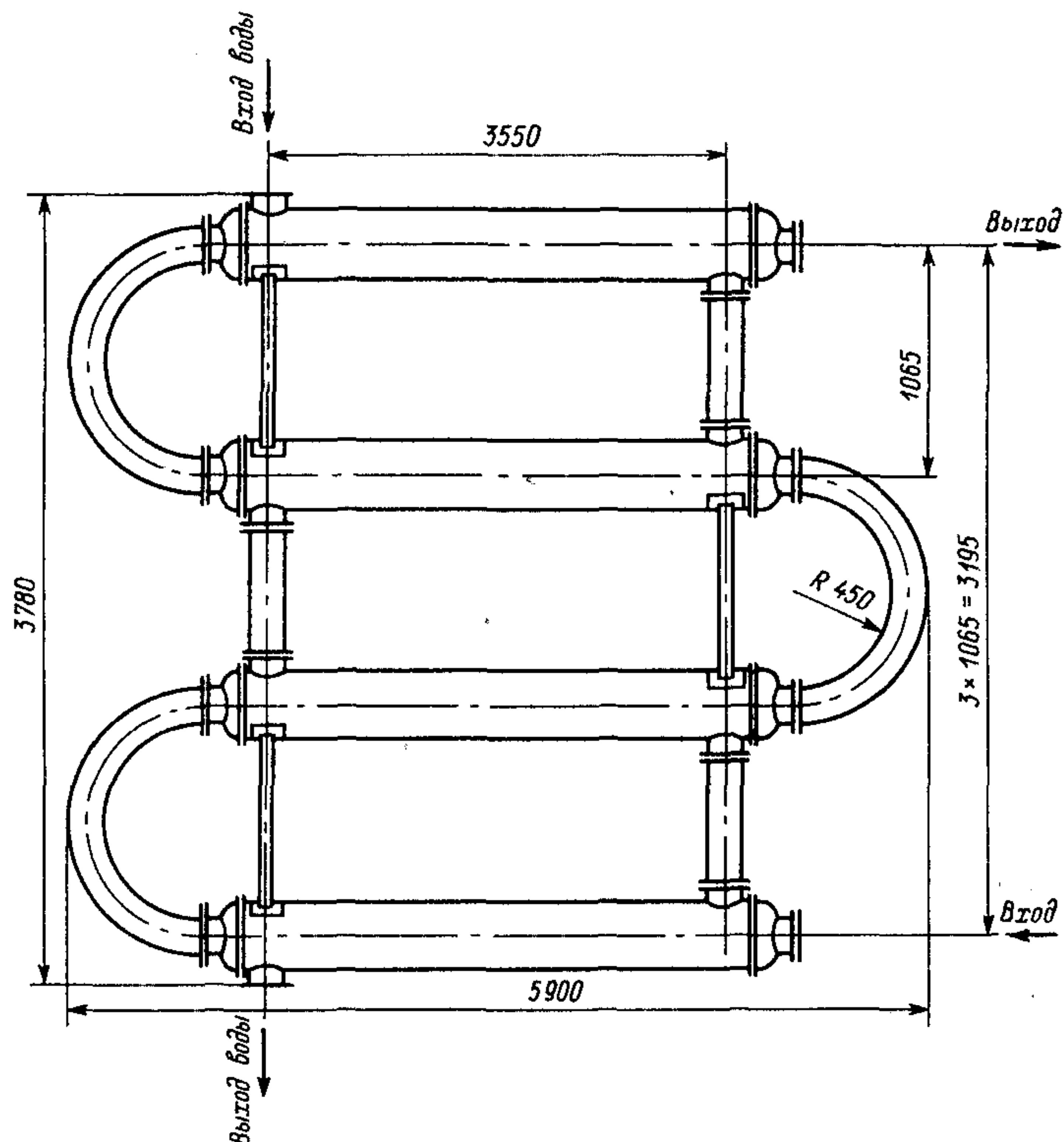
Рис. 5.14. Схема соединения теплообменников
