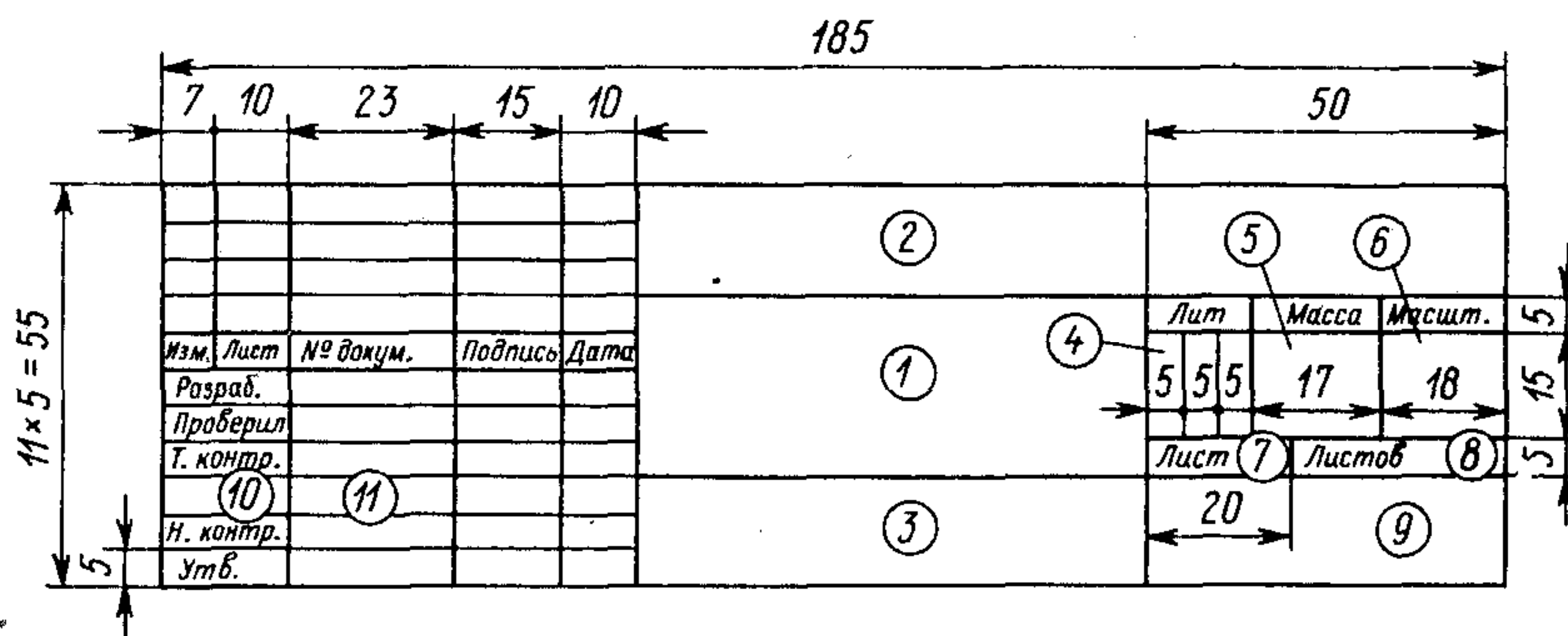
Рис. 12.6. Основная надпись на чертеже
