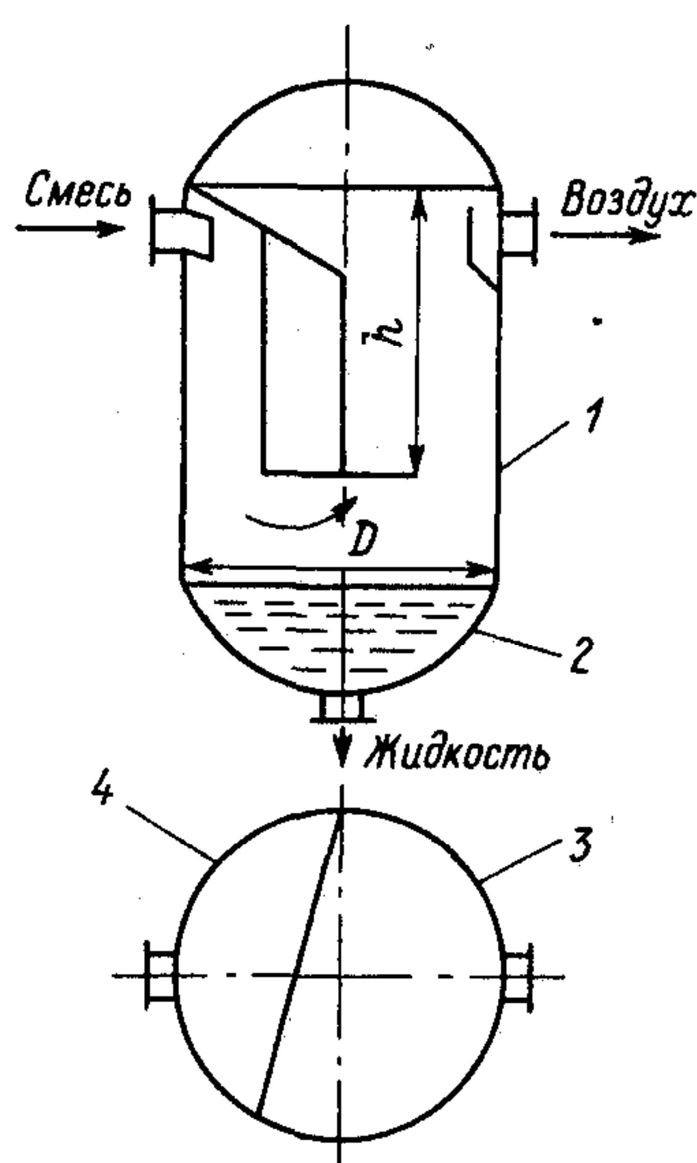
Рис. 4.3. Схема устройства ресивера:
