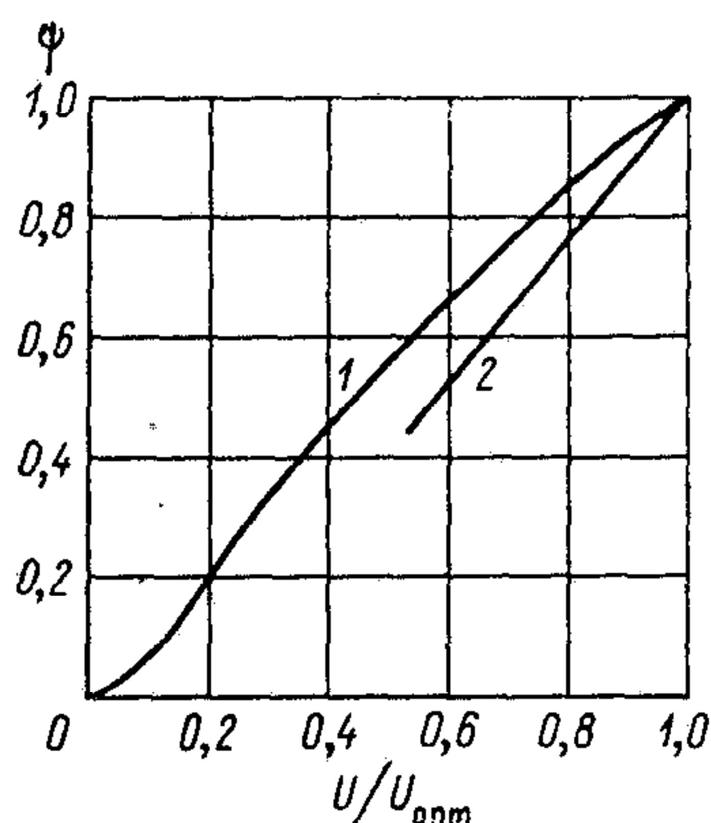
Рис. 8.5. Коэффициент смачиваемости \Psi при различном отношении U/U_{\text{опт}} : 1—на насадке из колец навалом; 2—на деревянной хордовой насадке
