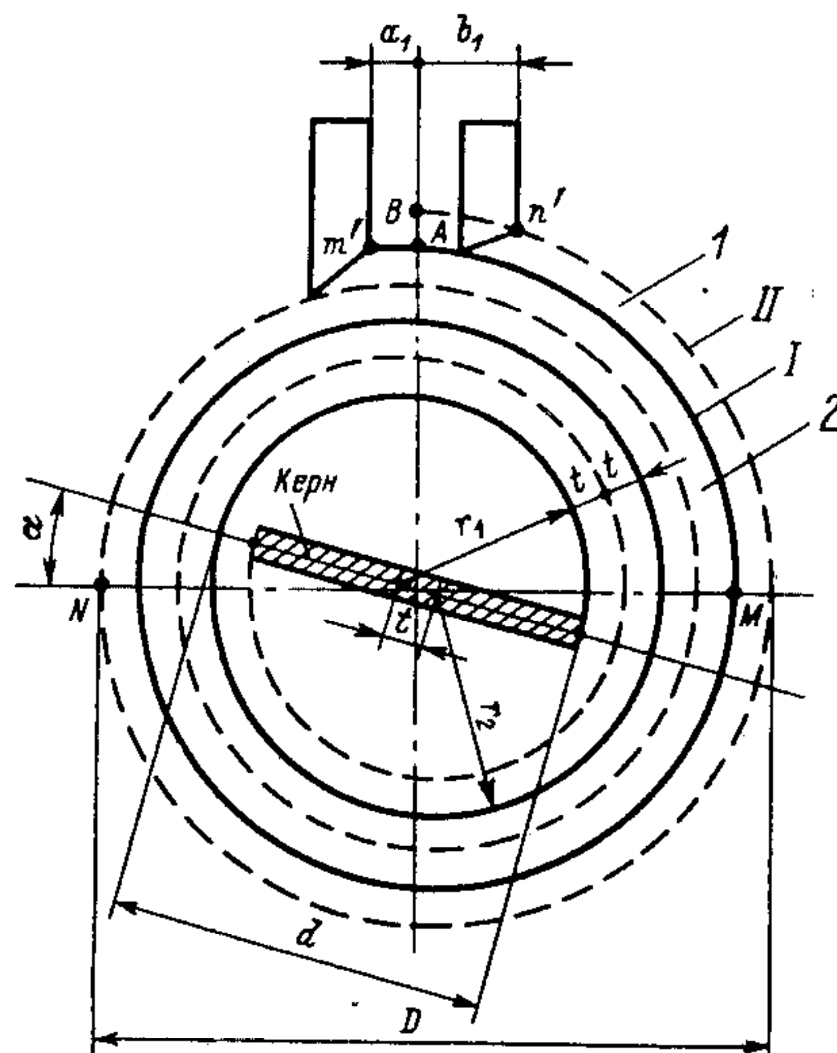
Рис. 5.7. Схема к расчету длины канала теплообменника:
